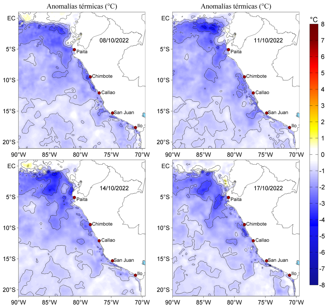
Figura 3. Anomalías de la temperatura superficial del mar (°C) para el 08, 11, 14 y 17 de octubre de 2022. Las anomalías se calcularon respecto de la climatología para el periodo 2007-2016. Datos: OSTIA-UKMO-L4-GLOB-v2.0 (UK Met Office, 2012; Donlon et al, 2012).
