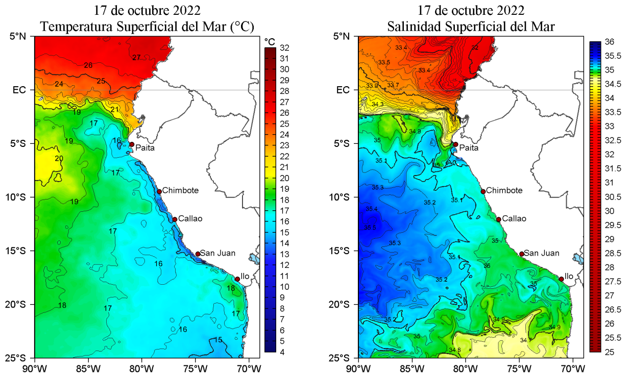
Figura 2. Temperatura superficial del mar (a la izquierda) y Salinidad superficial del mar (a la derecha) para el 17 de octubre de 2022. Datos: OSTIA-UKMO-L4-GLOB-v2.0 (UK Met Office, 2012; Donlon et al, 2012) y Hybrid Coordinate Ocean Model v. GOFS 3.1 (HYCOM; Halliwell et al., 1998; 2000; Bleck, 2001), respectivamente.
