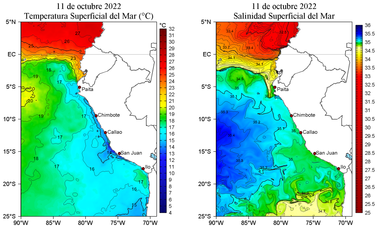
Figura 2. Temperatura superficial del mar (a la izquierda) y Salinidad superficial del mar (a la derecha) para el 11 de octubre de 2022. Datos: OSTIA-UKMO-L4-GLOB-v2.0 (UK Met Office, 2012; Donlon et al, 2012) y Hybrid Coordinate Ocean Model v. GOFS 3.1 (HYCOM; Halliwell et al., 1998; 2000; Bleck, 2001), respectivamente.
