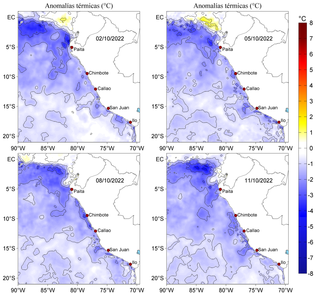
Figura 3. Anomalías de la temperatura superficial del mar (°C) para el 02, 05, 08 y 11 de octubre de 2022. Las anomalías se calcularon respecto de la climatología para el periodo 2007-2016. Datos: OSTIA-UKMO-L4-GLOB-v2.0 (UK Met Office, 2012; Donlon et al, 2012).
