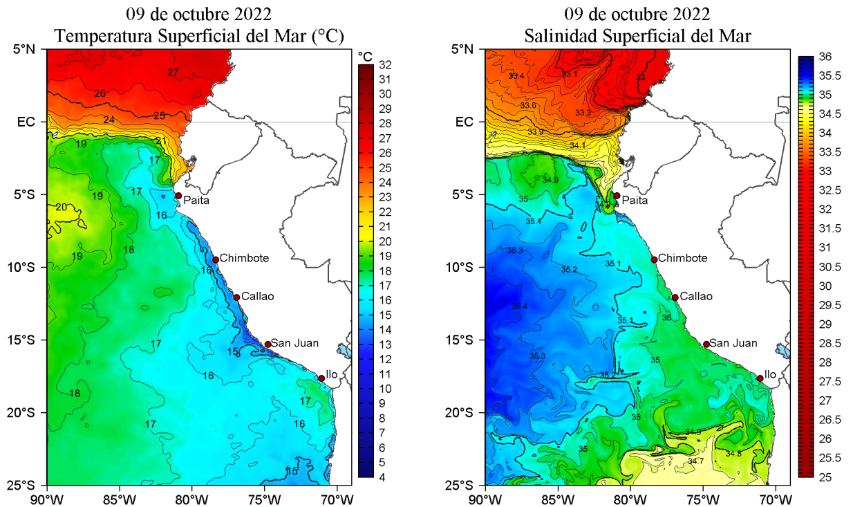
Figura 2. Temperatura superficial del mar (a la izquierda) y Salinidad superficial del mar (a la derecha) para el 09 de octubre de 2022. Datos: OSTIA-UKMO-L4-GLOB-v2.0 (UK Met Office, 2012; Donlon et al, 2012) y Hybrid Coordinate Ocean Model v. GOFS 3.1 (HYCOM; Halliwell et al., 1998; 2000; Bleck, 2001), respectivamente.
