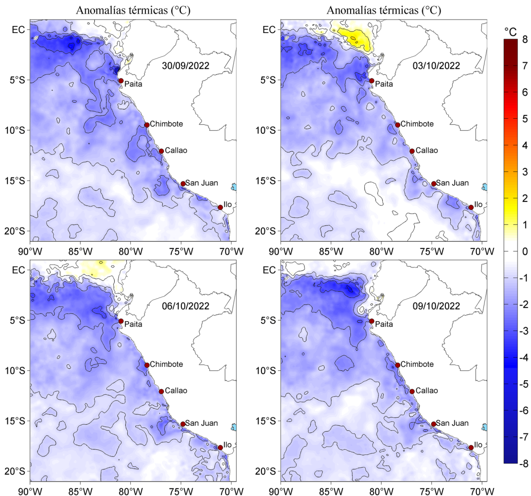
Figura 3. Anomalías de la temperatura superficial del mar (°C) para el 30 de setiembre, así como para el 03, 06 y 09 de octubre de 2022. Las anomalías se calcularon respecto de la climatología para el periodo 2007-2016. Datos: OSTIA-UKMO-L4-GLOB-v2.0 (UK Met Office, 2012; Donlon et al, 2012).
