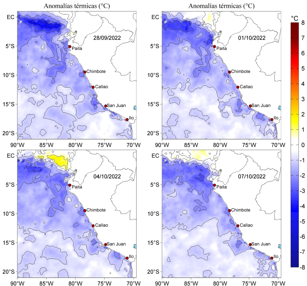
Figura 3. Anomalías de la temperatura superficial del mar (°C) para el 28 de setiembre, así como para el 01, 04 y 07 de octubre de 2022. Las anomalías se calcularon respecto de la climatología para el periodo 2007-2016. Datos: OSTIA-UKMO-L4-GLOB-v2.0 (UK Met Office, 2012; Donlon et al, 2012).
