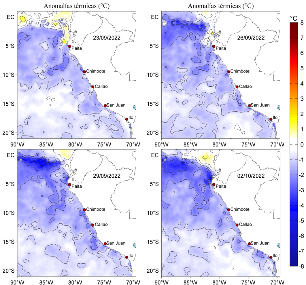
Figura 3. Anomalías de la temperatura superficial del mar (°C) para el 23, 26 y 29 de setiembre, así como para el 02 de octubre de 2022. Las anomalías se calcularon respecto de la climatología para el periodo 2007-2016. Datos: OSTIA-UKMO-L4-GLOB-v2.0 (UK Met Office, 2012; Donlon et al, 2012).
