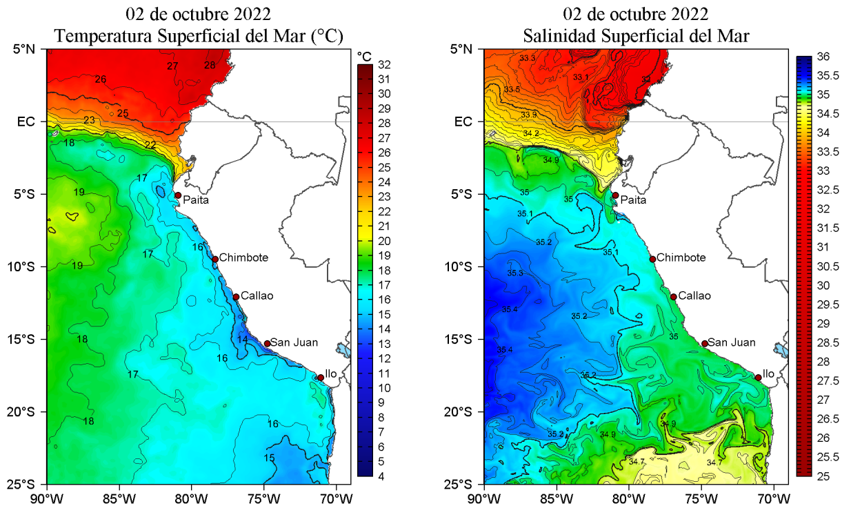
Figura 2. Temperatura superficial del mar (a la izquierda) y Salinidad superficial del mar (a la derecha) para el 02 de octubre de 2022. Datos: OSTIA-UKMO-L4-GLOB-v2.0 (UK Met Office, 2012; Donlon et al, 2012) y Hybrid Coordinate Ocean Model v. GOFS 3.1 (HYCOM; Halliwell et al., 1998; 2000; Bleck, 2001), respectivamente.
