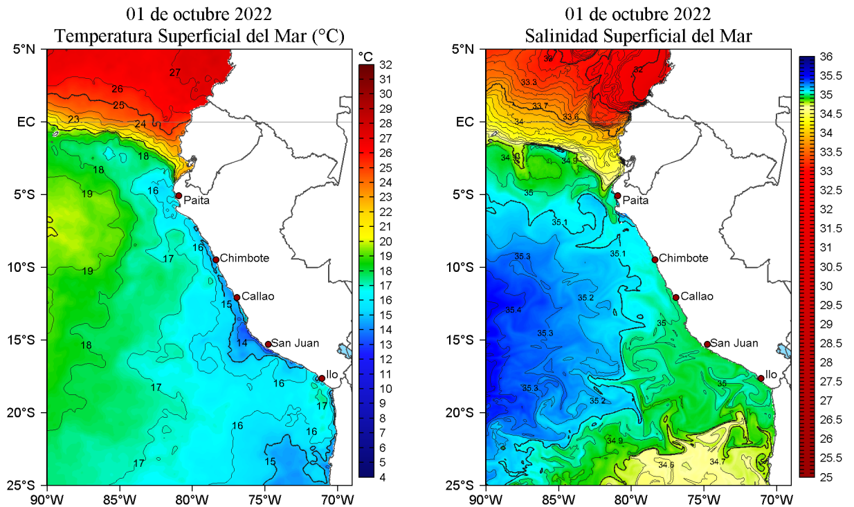
Figura 2. Temperatura superficial del mar (a la izquierda) y Salinidad superficial del mar (a la derecha) para el 01 de octubre de 2022. Datos: OSTIA-UKMO-L4-GLOB-v2.0 (UK Met Office, 2012; Donlon et al, 2012) y Hybrid Coordinate Ocean Model v. GOFS 3.1 (HYCOM; Halliwell et al., 1998; 2000; Bleck, 2001), respectivamente.
