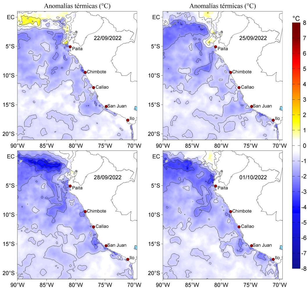
Figura 3. Anomalías de la temperatura superficial del mar (°C) para el 22, 25 y 28 de setiembre, así como para el 01 de octubre de 2022. Las anomalías se calcularon respecto de la climatología para el periodo 2007-2016. Datos: OSTIA-UKMO-L4-GLOB-v2.0 (UK Met Office, 2012; Donlon et al, 2012).
