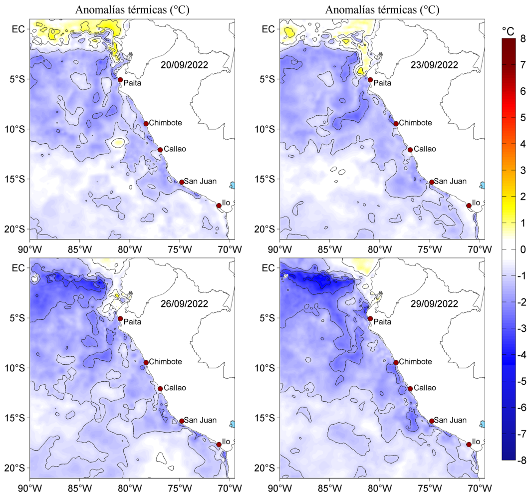
Figura 3. Anomalías de la temperatura superficial del mar (°C) para el 20, 23, 26 y 29 de setiembre de 2022. Las anomalías se calcularon respecto de la climatología para el periodo 2007-2016. Datos: OSTIA-UKMO-L4-GLOB-v2.0 (UK Met Office, 2012; Donlon et al, 2012).
