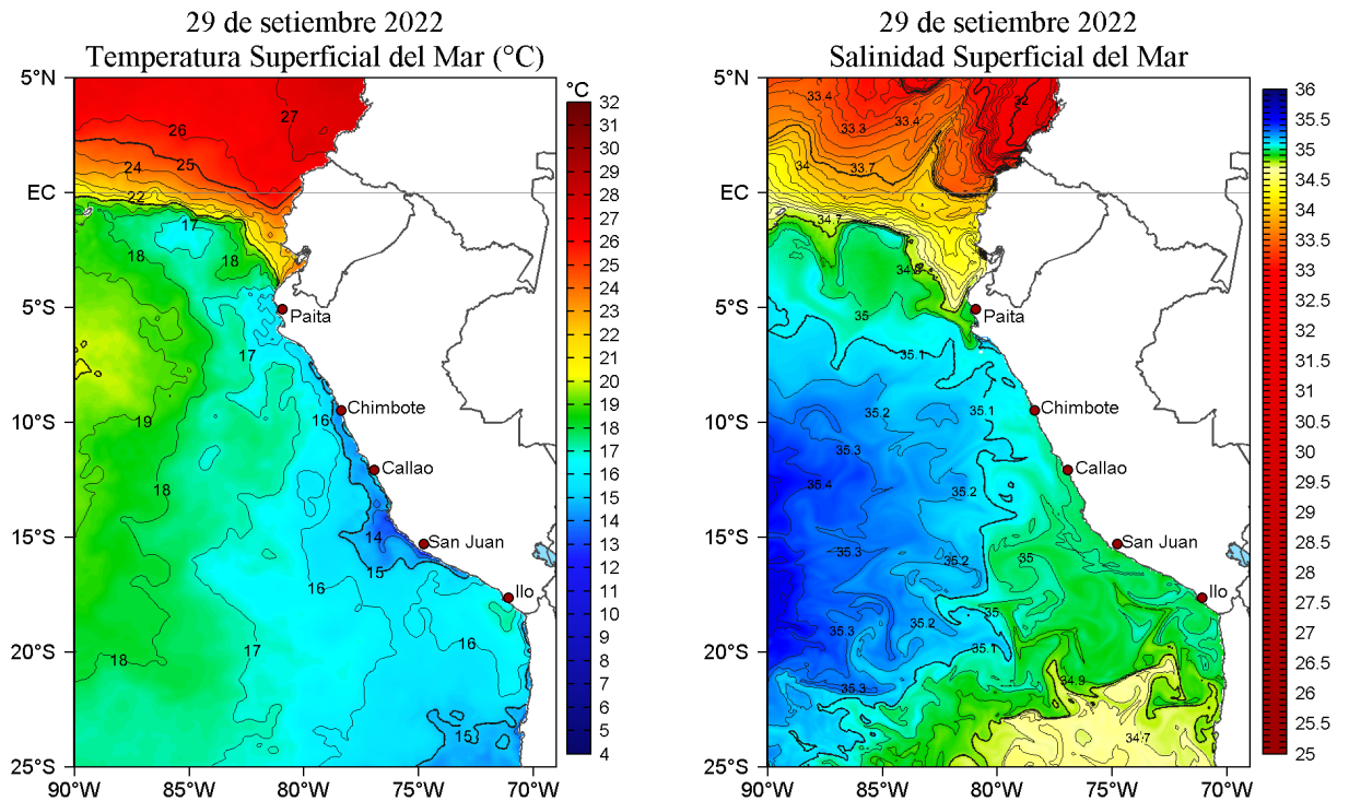
Figura 2. Temperatura superficial del mar (a la izquierda) y Salinidad superficial del mar (a la derecha) para el 29 de setiembre de 2022. Datos: OSTIA-UKMO-L4-GLOB-v2.0 (UK Met Office, 2012; Donlon et al, 2012) y Hybrid Coordinate Ocean Model v. GOFS 3.1 (HYCOM; Halliwell et al., 1998; 2000; Bleck, 2001), respectivamente.
