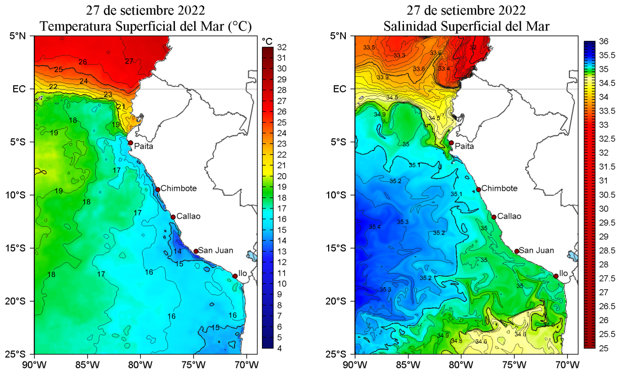
Figura 2. Temperatura superficial del mar (a la izquierda) y Salinidad superficial del mar (a la derecha) para el 27 de setiembre de 2022. Datos: OSTIA-UKMO-L4-GLOB-v2.0 (UK Met Office, 2012; Donlon et al, 2012) y Hybrid Coordinate Ocean Model v. GOFS 3.1 (HYCOM; Halliwell et al., 1998; 2000; Bleck, 2001), respectivamente.
