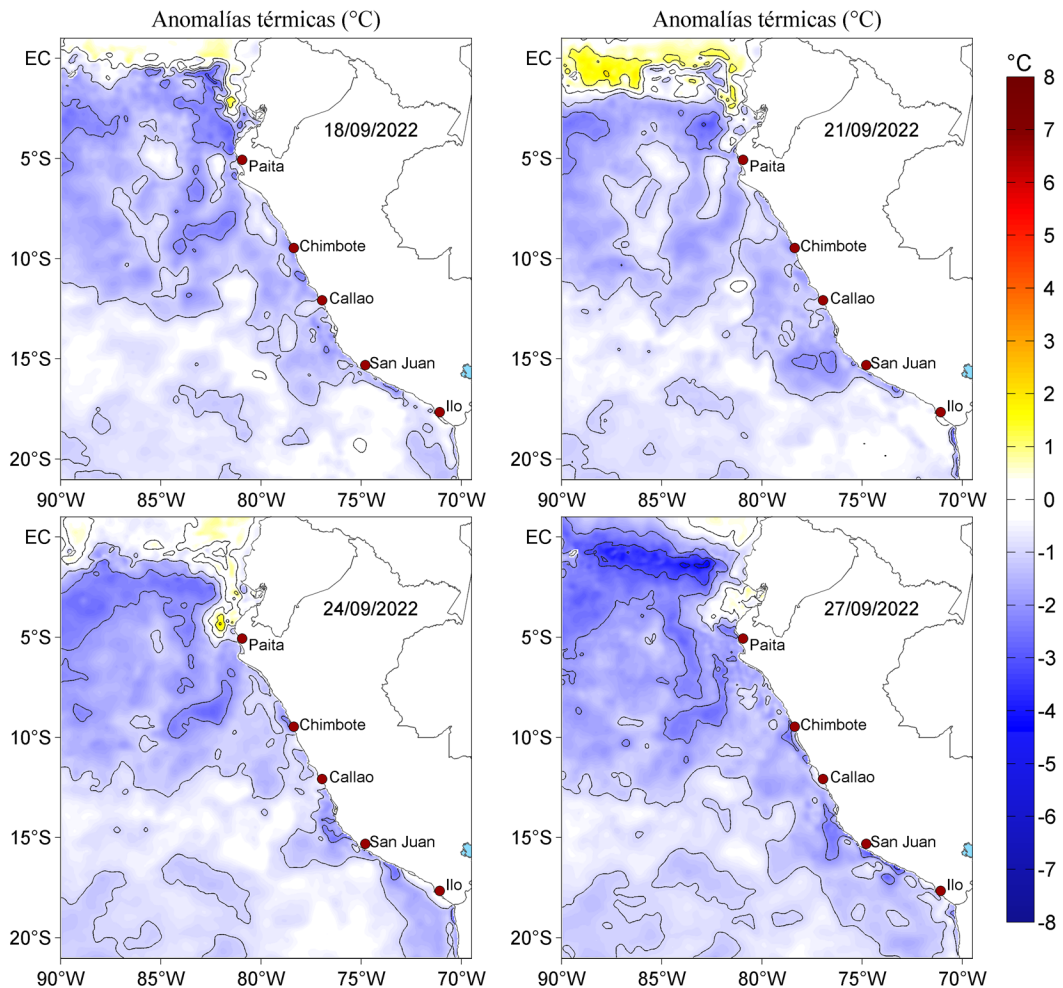
Figura 3. Anomalías de la temperatura superficial del mar (°C) para el 18, 21, 24 y 27 de setiembre de 2022. Las anomalías se calcularon respecto de la climatología para el periodo 2007-2016. Datos: OSTIA-UKMO-L4-GLOB-v2.0 (UK Met Office, 2012; Donlon et al, 2012).
