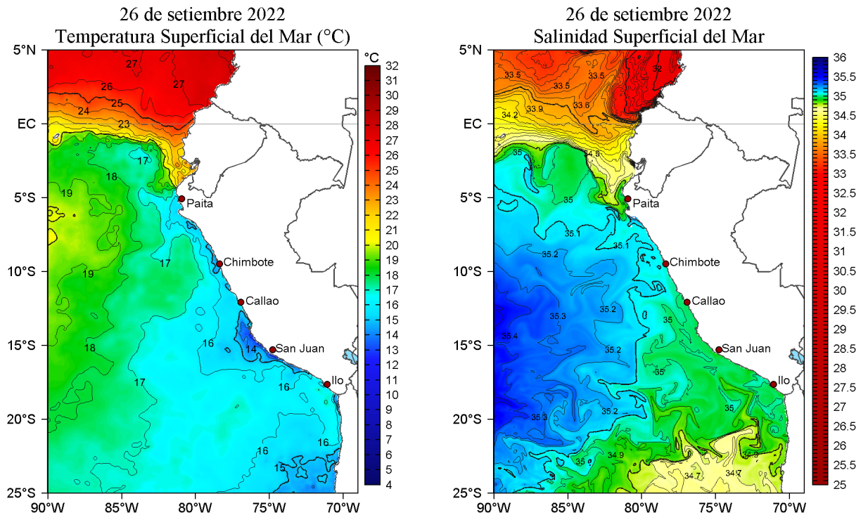
Figura 2. Temperatura superficial del mar (a la izquierda) y Salinidad superficial del mar (a la derecha) para el 26 de setiembre de 2022. Datos: OSTIA-UKMO-L4-GLOB-v2.0 (UK Met Office, 2012; Donlon et al, 2012) y Hybrid Coordinate Ocean Model v. GOFS 3.1 (HYCOM; Halliwell et al., 1998; 2000; Bleck, 2001), respectivamente.
