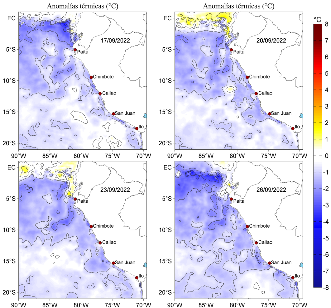
Figura 3. Anomalías de la temperatura superficial del mar (°C) para el 17, 20, 23 y 26 de setiembre de 2022. Las anomalías se calcularon respecto de la climatología para el periodo 2007-2016. Datos: OSTIA-UKMO-L4-GLOB-v2.0 (UK Met Office, 2012; Donlon et al, 2012).
