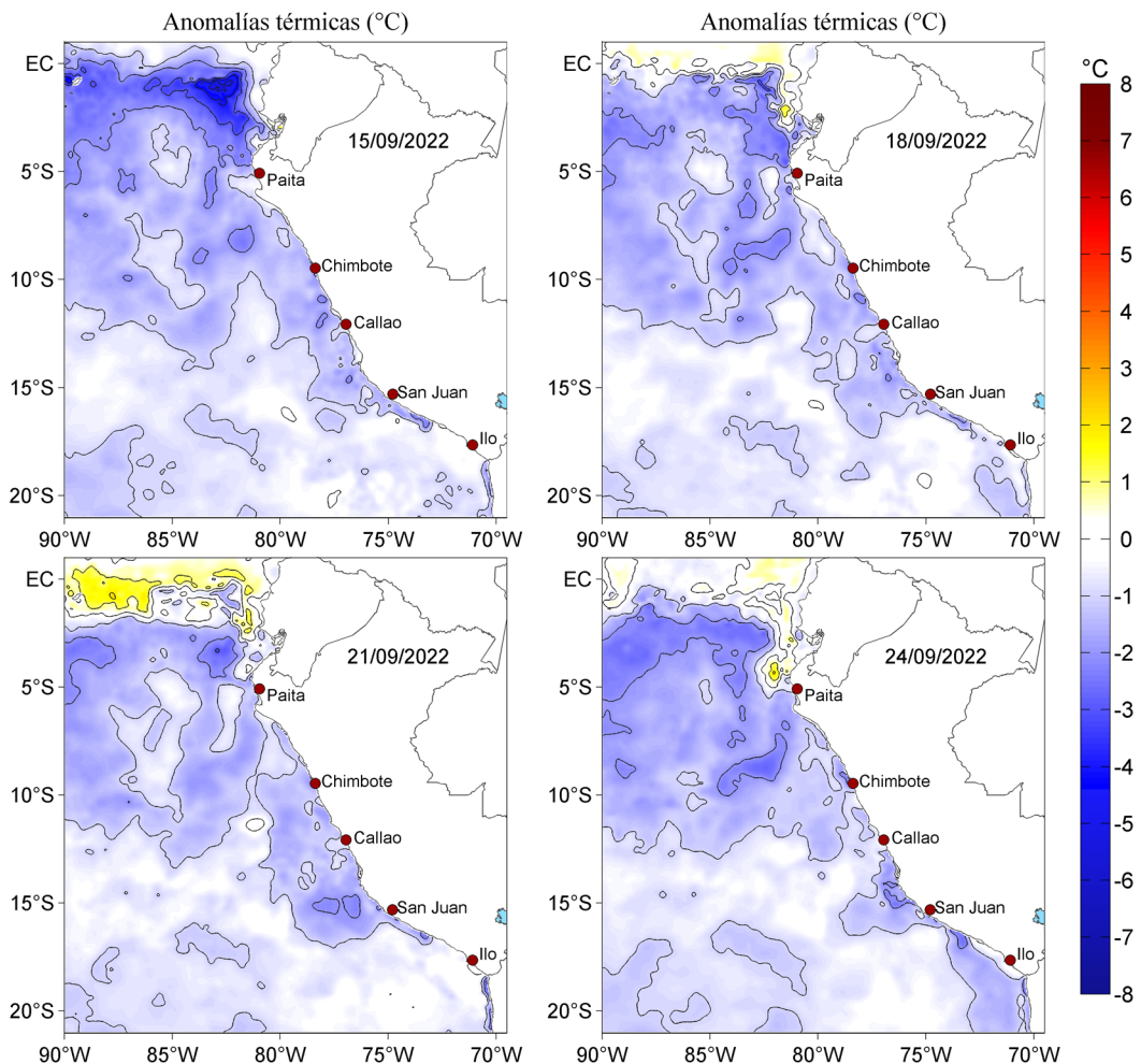
Figura 3. Anomalías de la temperatura superficial del mar (°C) para el 15, 18, 21 y 24 de setiembre de 2022. Las anomalías se calcularon respecto de la climatología para el periodo 2007-2016. Datos: OSTIA-UKMO-L4-GLOB-v2.0 (UK Met Office, 2012; Donlon et al, 2012).
