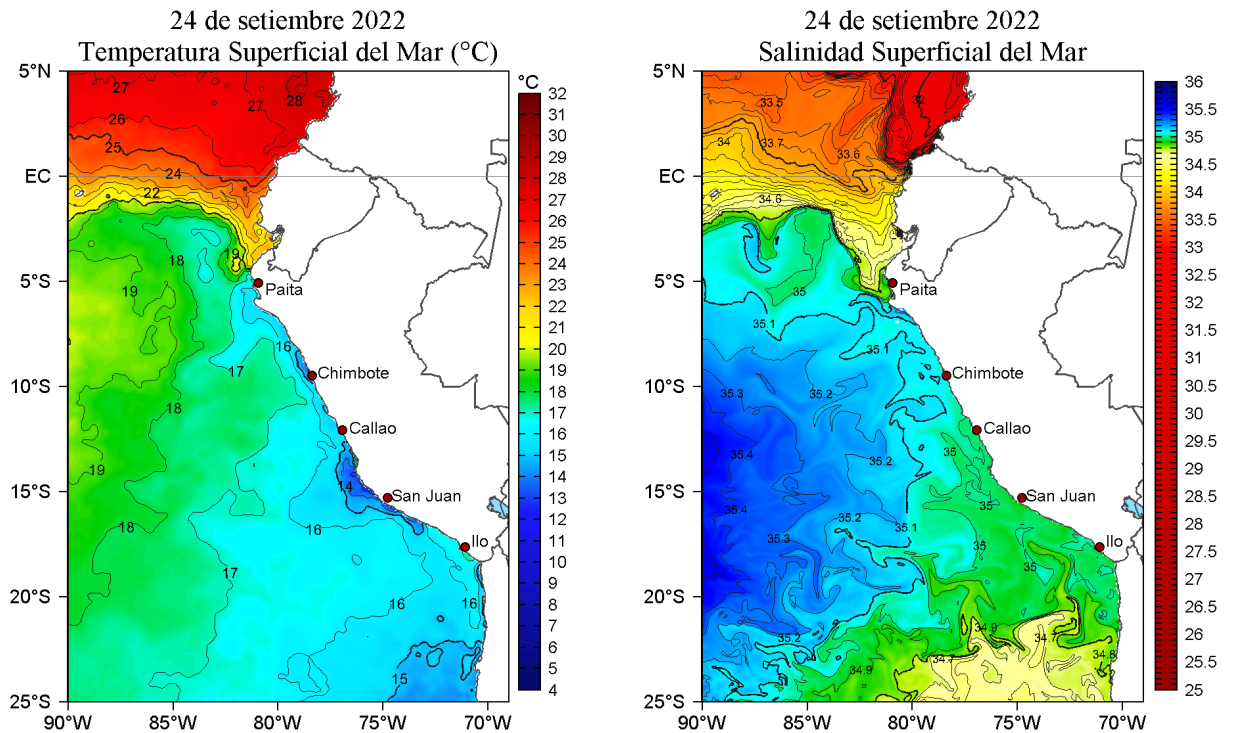
Figura 2. Temperatura superficial del mar (a la izquierda) y Salinidad superficial del mar (a la derecha) para el 24 de setiembre de 2022. Datos: OSTIA-UKMO-L4-GLOB-v2.0 (UK Met Office, 2012; Donlon et al, 2012) y Hybrid Coordinate Ocean Model v. GOFS 3.1 (HYCOM; Halliwell et al., 1998; 2000; Bleck, 2001), respectivamente.
