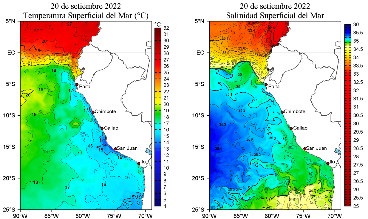
Figura 2. Temperatura superficial del mar (a la izquierda) y Salinidad superficial del mar (a la derecha) para el 20 de setiembre de 2022. Datos: OSTIA-UKMO-L4-GLOB-v2.0 (UK Met Office, 2012; Donlon et al, 2012) y Hybrid Coordinate Ocean Model v. GOFS 3.1 (HYCOM; Halliwell et al., 1998; 2000; Bleck, 2001), respectivamente.
