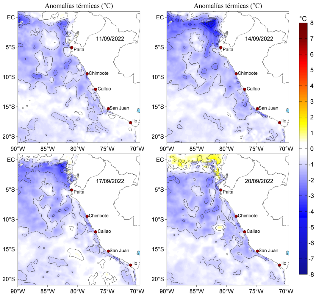
Figura 3. Anomalías de la temperatura superficial del mar (°C) para el 11, 14, 17 y 20 de setiembre de 2022. Las anomalías se calcularon respecto de la climatología para el periodo 2007-2016. Datos: OSTIA-UKMO-L4-GLOB-v2.0 (UK Met Office, 2012; Donlon et al, 2012).
