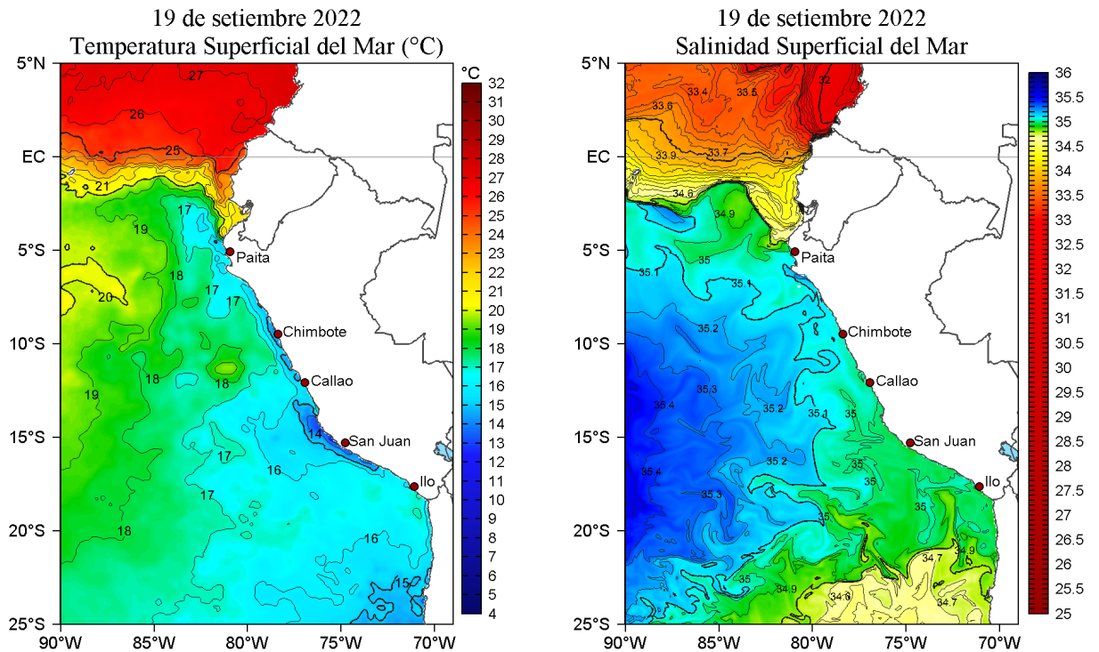
Figura 2. Temperatura superficial del mar (a la izquierda) y Salinidad superficial del mar (a la derecha) para el 19 de setiembre de 2022. Datos: OSTIA-UKMO-L4-GLOB-v2.0 (UK Met Office, 2012; Donlon et al, 2012) y Hybrid Coordinate Ocean Model v. GOFS 3.1 (HYCOM; Halliwell et al., 1998; 2000; Bleck, 2001), respectivamente.
