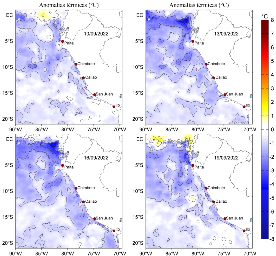
Figura 3. Anomalías de la temperatura superficial del mar (°C) para el 10, 13, 16 y 19 de setiembre de 2022. Las anomalías se calcularon respecto de la climatología para el periodo 2007-2016. Datos: OSTIA-UKMO-L4-GLOB-v2.0 (UK Met Office, 2012; Donlon et al, 2012).
