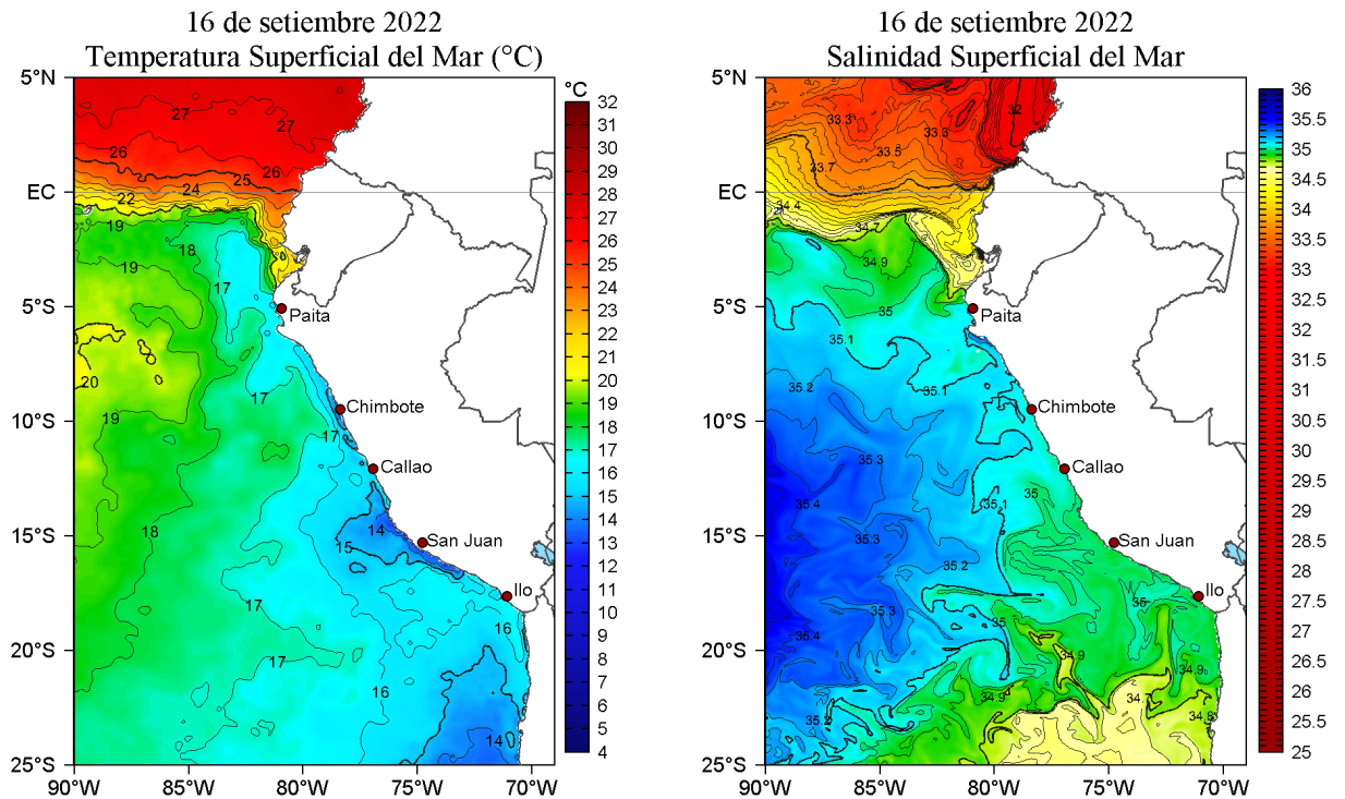
Figura 2. Temperatura superficial del mar (a la izquierda) y Salinidad superficial del mar (a la derecha) para el 16 de setiembre de 2022. Datos: OSTIA-UKMO-L4-GLOB-v2.0 (UK Met Office, 2012; Donlon et al, 2012) y Hybrid Coordinate Ocean Model v. GOFS 3.1 (HYCOM; Halliwell et al., 1998; 2000; Bleck, 2001), respectivamente.
