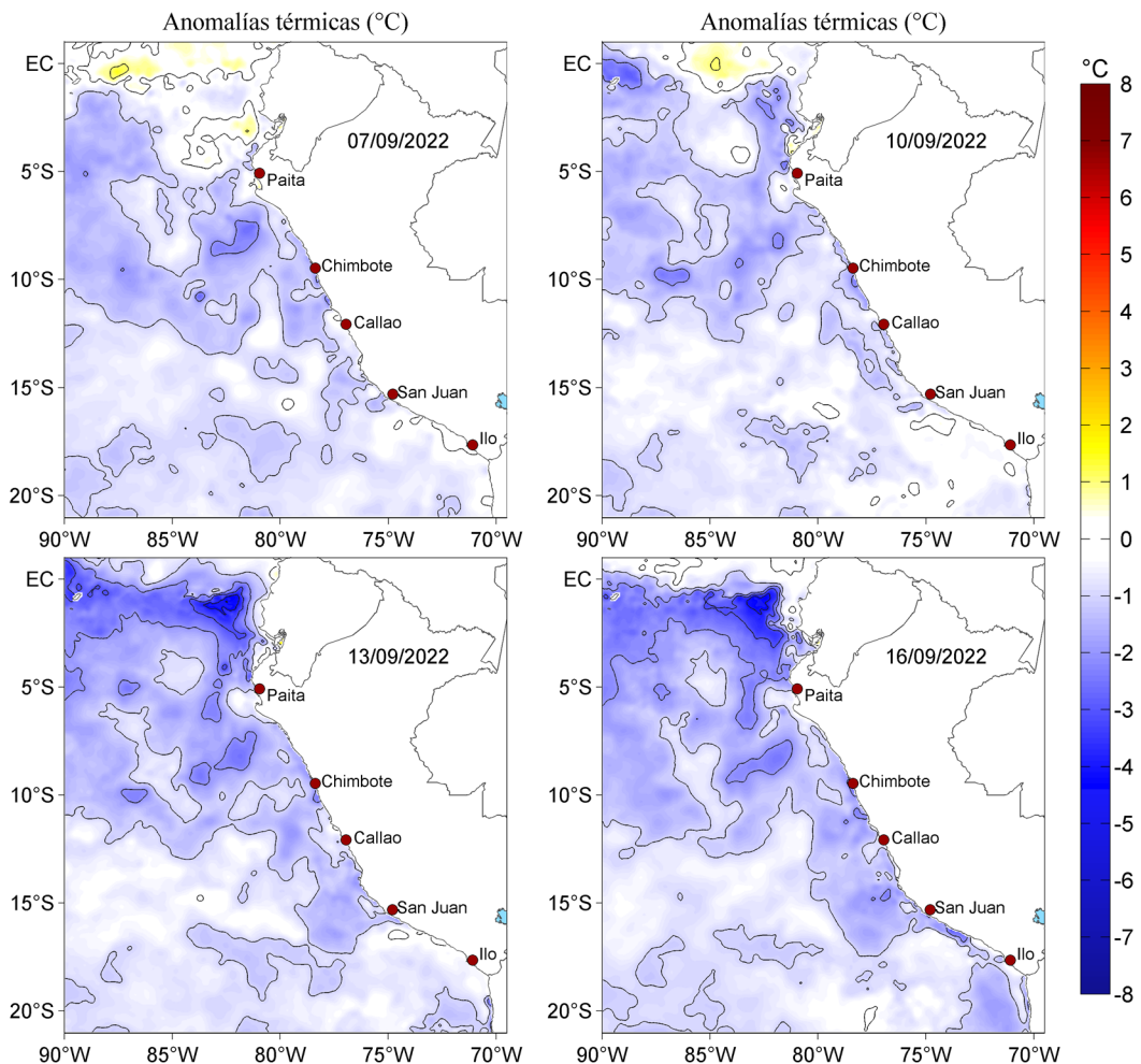
Figura 3. Anomalías de la temperatura superficial del mar (°C) para el 07, 10, 13 y 16 de setiembre de 2022. Las anomalías se calcularon respecto de la climatología para el periodo 2007-2016. Datos: OSTIA-UKMO-L4-GLOB-v2.0 (UK Met Office, 2012; Donlon et al, 2012).
