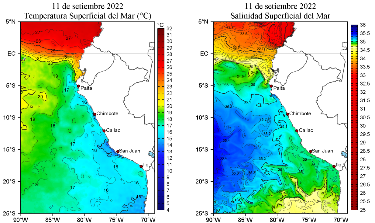
Figura 2. Temperatura superficial del mar (a la izquierda) y Salinidad superficial del mar (a la derecha) para el 11 de setiembre de 2022. Datos: OSTIA-UKMO-L4-GLOB-v2.0 (UK Met Office, 2012; Donlon et al, 2012) y Hybrid Coordinate Ocean Model v. GOFS 3.1 (HYCOM; Halliwell et al., 1998; 2000; Bleck, 2001), respectivamente.
