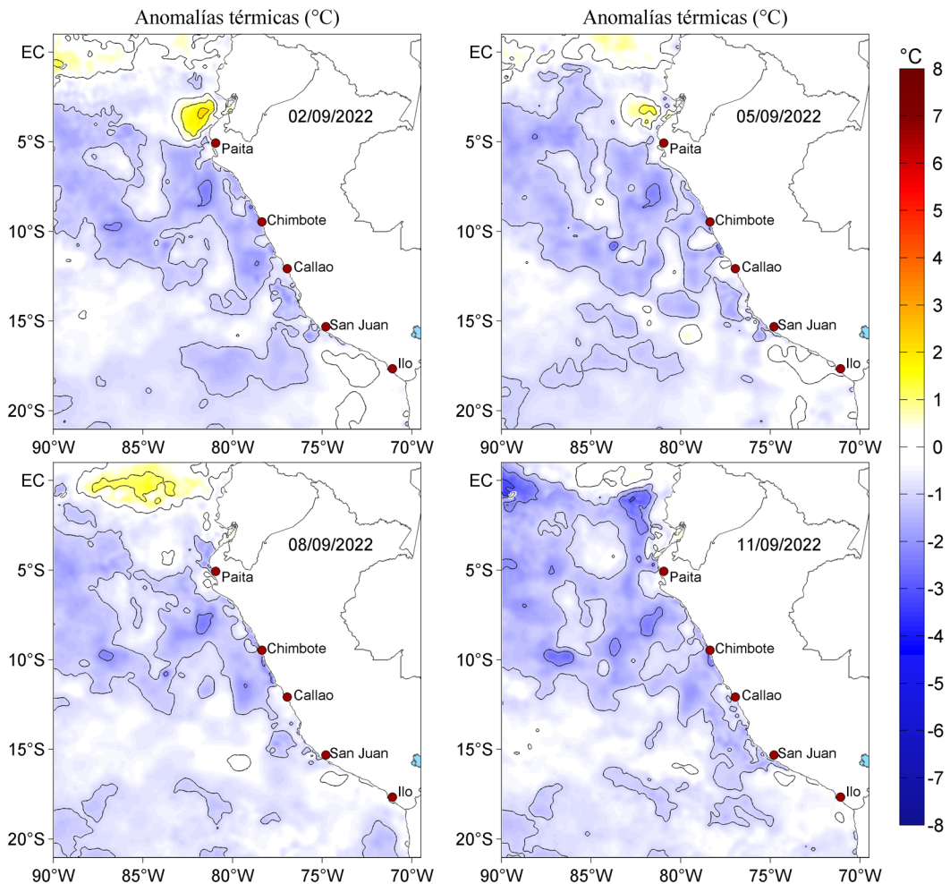
Figura 3. Anomalías de la temperatura superficial del mar (°C) para el 02, 05, 08 y 11 de setiembre de 2022. Las anomalías se calcularon respecto de la climatología para el periodo 2007-2016. Datos: OSTIA-UKMO-L4-GLOB-v2.0 (UK Met Office, 2012; Donlon et al, 2012).
