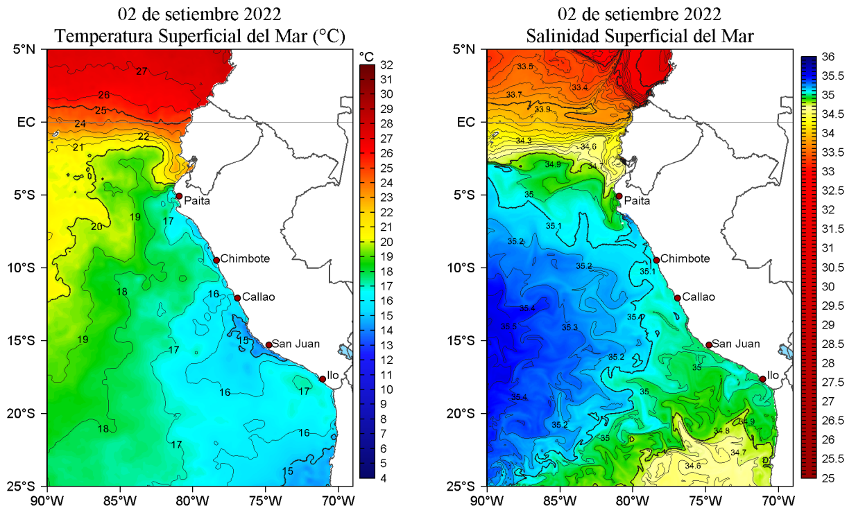
Figura 2. Temperatura superficial del mar (a la izquierda) y Salinidad superficial del mar (a la derecha) para el 02 de setiembre de 2022. Datos: OSTIA-UKMO-L4-GLOB-v2.0 (UK Met Office, 2012; Donlon et al, 2012) y Hybrid Coordinate Ocean Model v. GOFS 3.1 (HYCOM; Halliwell et al., 1998; 2000; Bleck, 2001), respectivamente.
