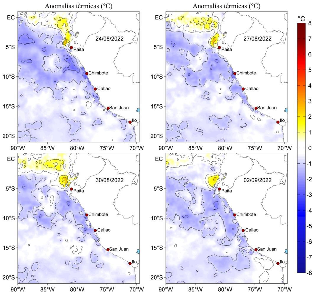
Figura 3. Anomalías de la temperatura superficial del mar (°C) para el 24, 27 y 30 de agosto, así como para el 02 de setiembre de 2022. Las anomalías se calcularon respecto de la climatología para el periodo 2007-2016. Datos: OSTIA-UKMO-L4-GLOB-v2.0 (UK Met Office, 2012; Donlon et al, 2012).
