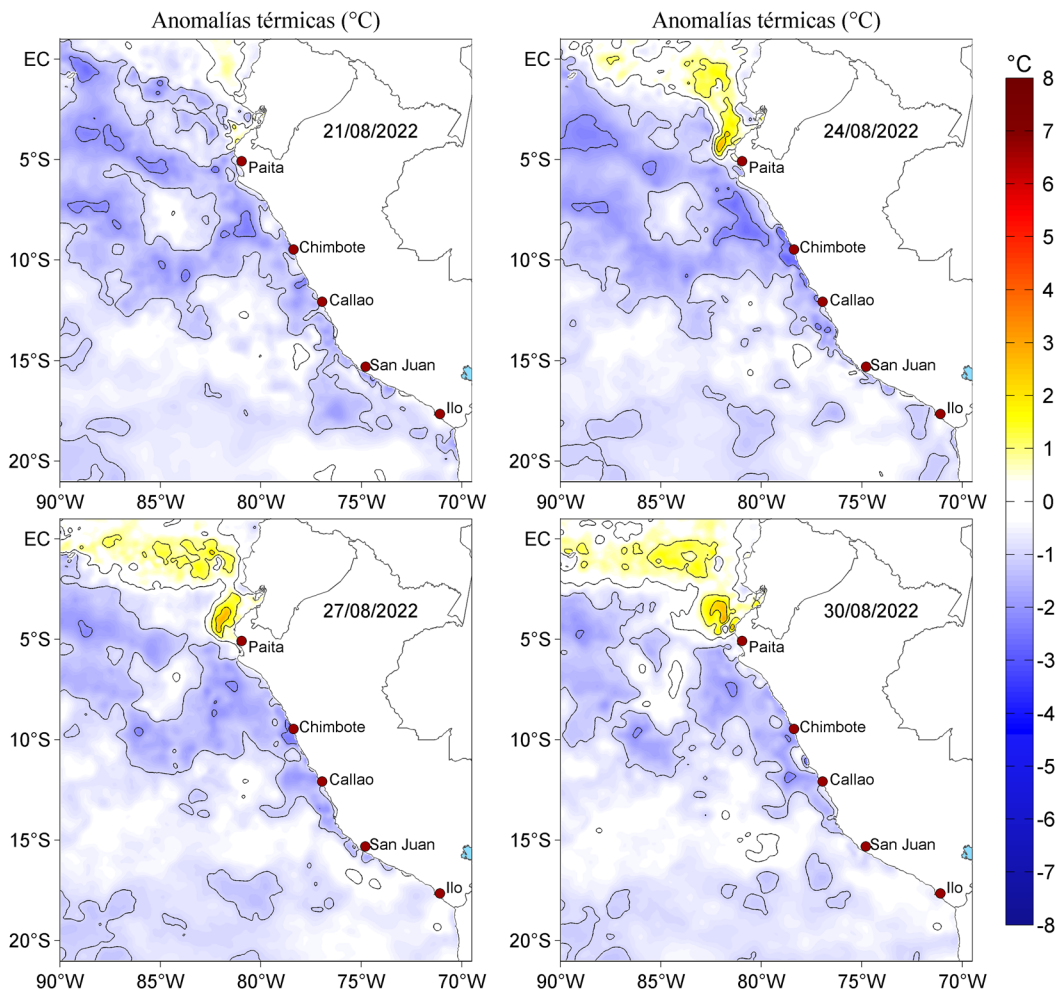
Figura 3. Anomalías de la temperatura superficial del mar (°C) para el 21, 24, 27 y 30 de agosto de 2022. Las anomalías se calcularon respecto de la climatología para el periodo 2007-2016. Datos: OSTIA-UKMO-L4-GLOB-v2.0 (UK Met Office, 2012; Donlon et al, 2012).
