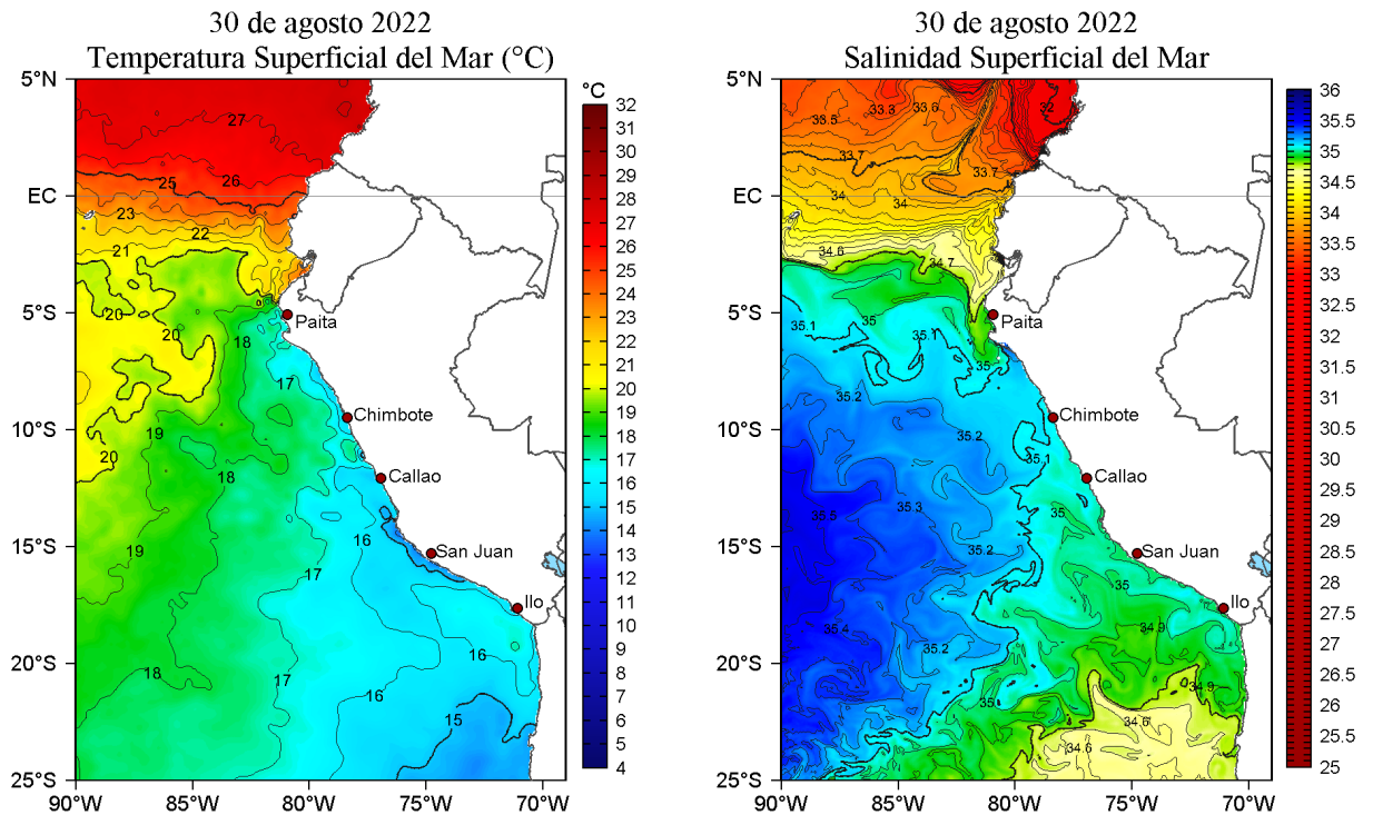
Figura 2. Temperatura superficial del mar (a la izquierda) y Salinidad superficial del mar (a la derecha) para el 30 de agosto de 2022. Datos: OSTIA-UKMO-L4-GLOB-v2.0 (UK Met Office, 2012; Donlon et al, 2012) y Hybrid Coordinate Ocean Model v. GOFS 3.1 (HYCOM; Halliwell et al., 1998; 2000; Bleck, 2001), respectivamente.
