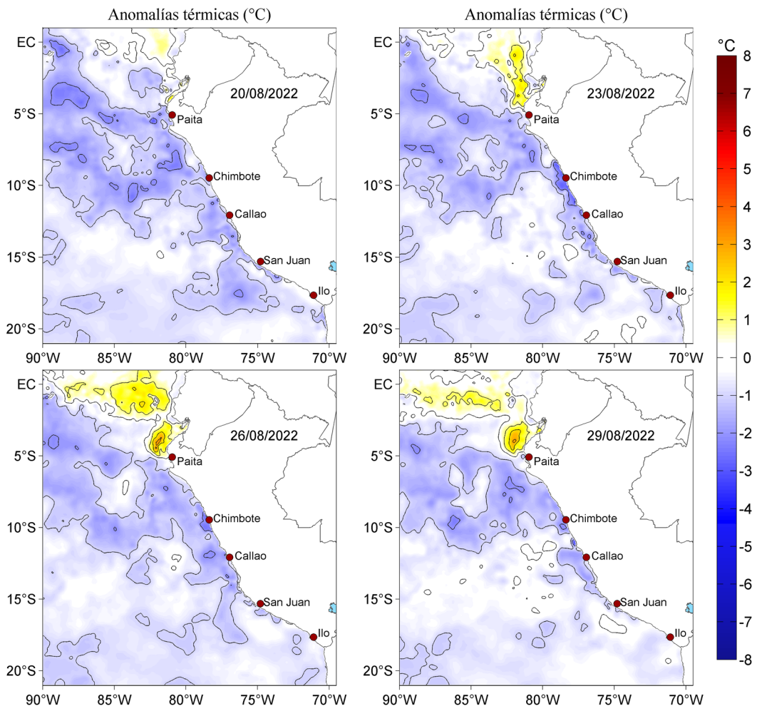
Figura 3. Anomalías de la temperatura superficial del mar ( ^{\circ}\text{C} ) para el 20, 23, 26 y 29 de agosto de 2022. Las anomalías se calcularon respecto de la climatología para el periodo 2007-2016. Datos: OSTIA-UKMO-L4-GLOB-v2.0 (UK Met Office, 2012; Donlon et al, 2012).
