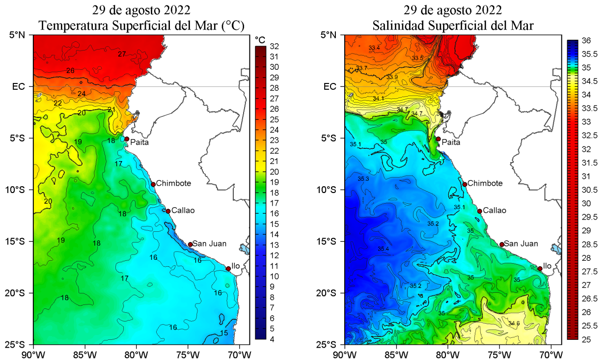
Figura 2. Temperatura superficial del mar (a la izquierda) y Salinidad superficial del mar (a la derecha) para el 29 de agosto de 2022. Datos: OSTIA-UKMO-L4-GLOB-v2.0 (UK Met Office, 2012; Donlon et al, 2012) y Hybrid Coordinate Ocean Model v. GOFS 3.1 (HYCOM; Halliwell et al., 1998; 2000; Bleck, 2001), respectivamente.
