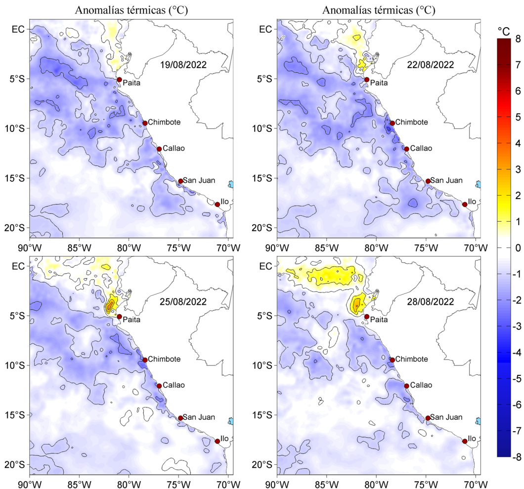
Figura 3. Anomalías de la temperatura superficial del mar (°C) para el 19, 22, 25 y 28 de agosto de 2022. Las anomalías se calcularon respecto de la climatología para el periodo 2007-2016. Datos: OSTIA-UKMO-L4-GLOB-v2.0 (UK Met Office, 2012; Donlon et al, 2012).
