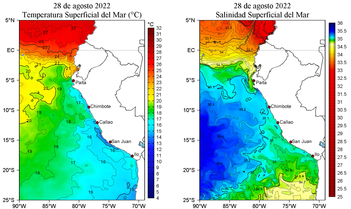
Figura 2. Temperatura superficial del mar (a la izquierda) y Salinidad superficial del mar (a la derecha) para el 28 de agosto de 2022. Datos: OSTIA-UKMO-L4-GLOB-v2.0 (UK Met Office, 2012; Donlon et al, 2012) y Hybrid Coordinate Ocean Model v. GOFS 3.1 (HYCOM; Halliwell et al., 1998; 2000; Bleck, 2001), respectivamente.
