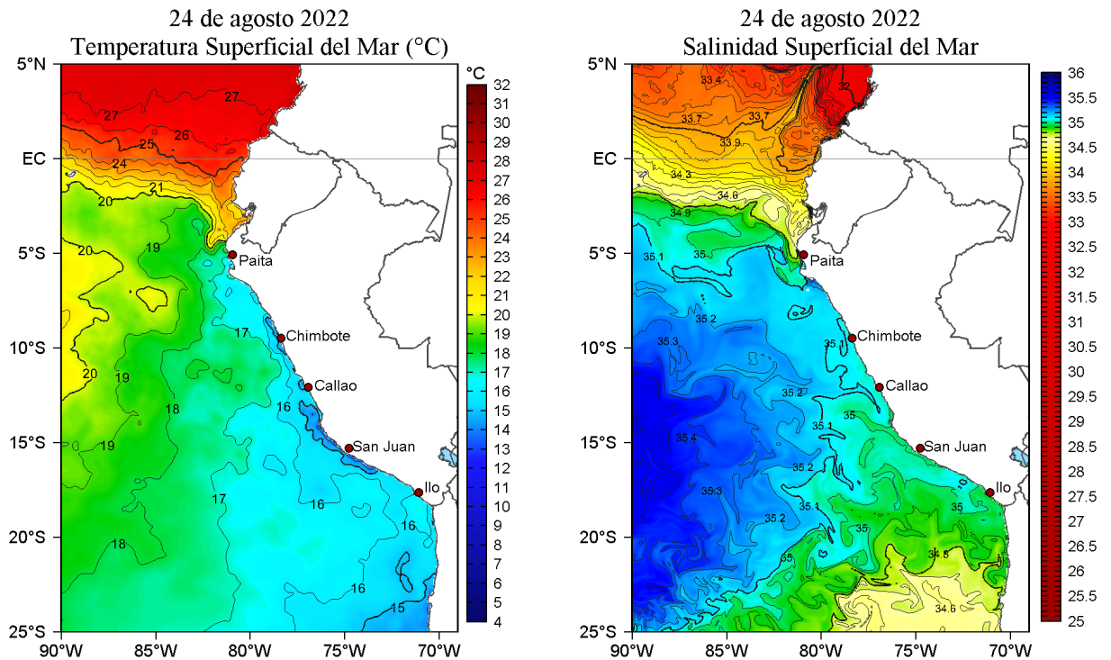
Figura 2. Temperatura superficial del mar (a la izquierda) y Salinidad superficial del mar (a la derecha) para el 24 de agosto de 2022. Datos: OSTIA-UKMO-L4-GLOB-v2.0 (UK Met Office, 2012; Donlon et al, 2012) y Hybrid Coordinate Ocean Model v. GOFS 3.1 (HYCOM; Halliwell et al., 1998; 2000; Bleck, 2001), respectivamente.
