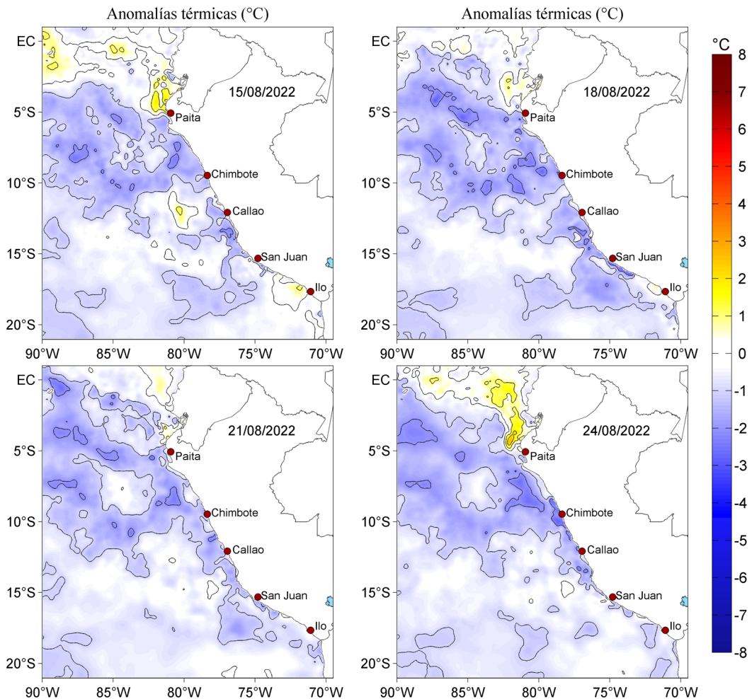
Figura 3. Anomalías de la temperatura superficial del mar (°C) para el 15, 18, 21 y 24 de agosto de 2022. Las anomalías se calcularon respecto de la climatología para el periodo 2007-2016. Datos: OSTIA-UKMO-L4-GLOB-v2.0 (UK Met Office, 2012; Donlon et al, 2012).
