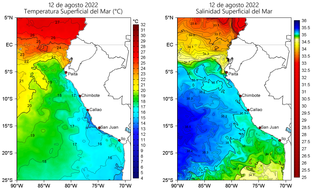
Figura 2. Temperatura superficial del mar (a la izquierda) y Salinidad superficial del mar (a la derecha) para el 12 de agosto de 2022. Datos: OSTIA-UKMO-L4-GLOB-v2.0 (UK Met Office, 2012; Donlon et al, 2012) y Hybrid Coordinate Ocean Model v. GOFS 3.1 (HYCOM; Halliwell et al., 1998; 2000; Bleck, 2001), respectivamente.
