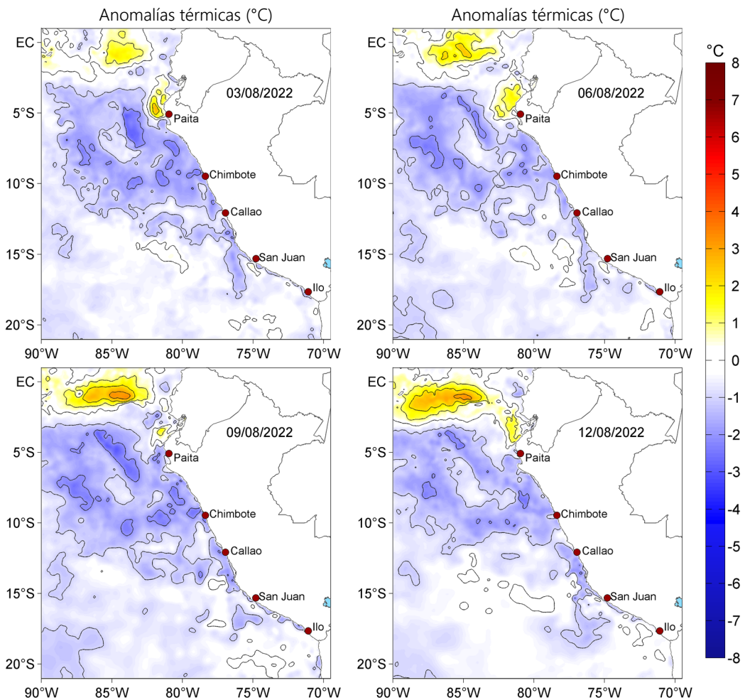
Figura 3. Anomalías de la temperatura superficial del mar (°C) para el 03, 06, 09 y 12 de agosto de 2022. Las anomalías se calcularon respecto de la climatología para el periodo 2007-2016. Datos: OSTIA-UKMO-L4-GLOB-v2.0 (UK Met Office, 2012; Donlon et al, 2012).
