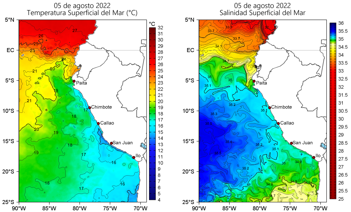
Figura 2. Temperatura superficial del mar (a la izquierda) y Salinidad superficial del mar (a la derecha) para el 05 de agosto de 2022. Datos: OSTIA-UKMO-L4-GLOB-v2.0 (UK Met Office, 2012; Donlon et al, 2012) y Hybrid Coordinate Ocean Model v. GOFS 3.1 (HYCOM; Halliwell et al., 1998; 2000; Bleck, 2001), respectivamente.
