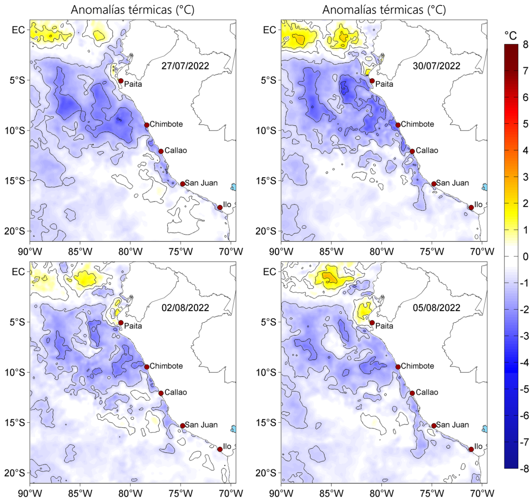
Figura 3. Anomalías de la temperatura superficial del mar (°C) para el 27 y 30 de julio, así como para el 02 y 05 de agosto de 2022. Las anomalías se calcularon respecto de la climatología para el periodo 2007-2016. Datos: OSTIA-UKMO-L4-GLOB-v2.0 (UK Met Office, 2012; Donlon et al, 2012).
