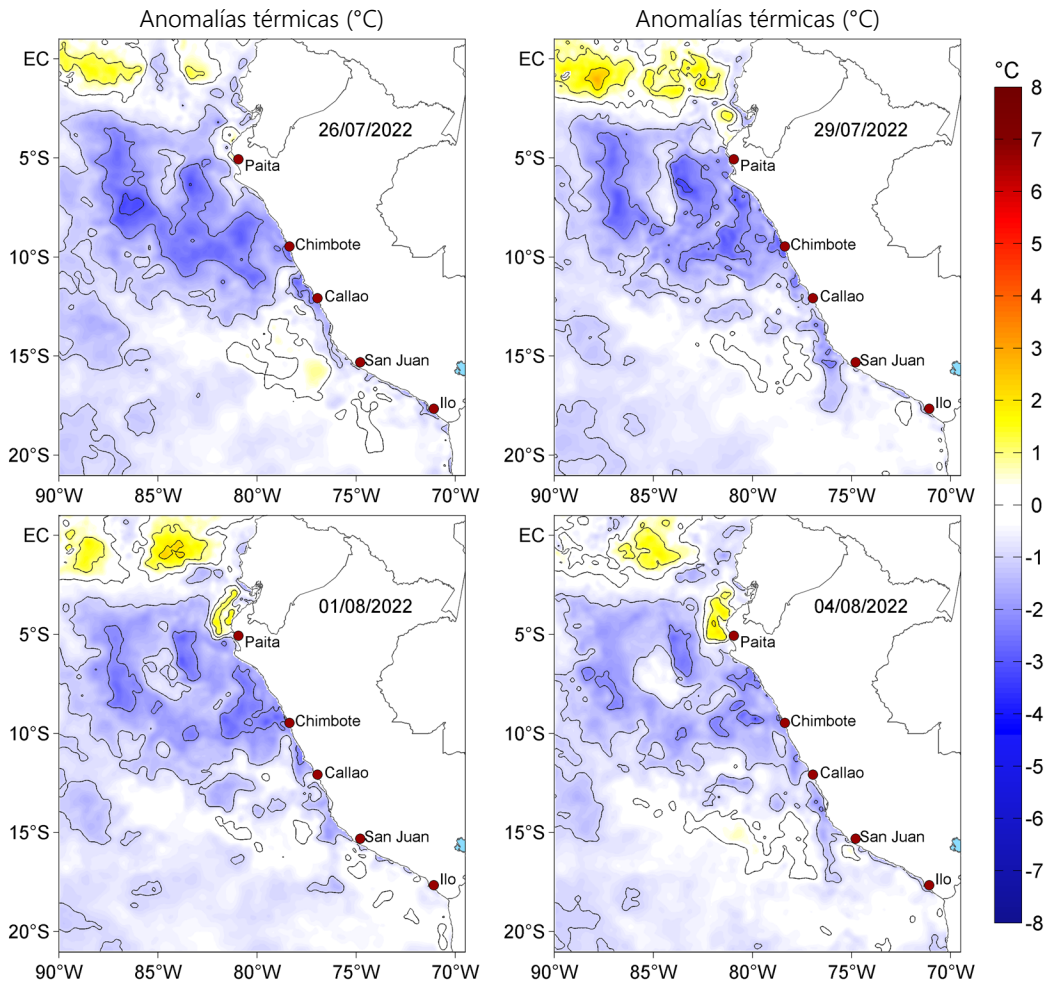
Figura 3. Anomalías de la temperatura superficial del mar (°C) para el 26 y 29 de julio, así como para el 01 y 04 de agosto de 2022. Las anomalías se calcularon respecto de la climatología para el periodo 2007-2016. Datos: OSTIA-UKMO-L4-GLOB-v2.0 (UK Met Office, 2012; Donlon et al, 2012).
