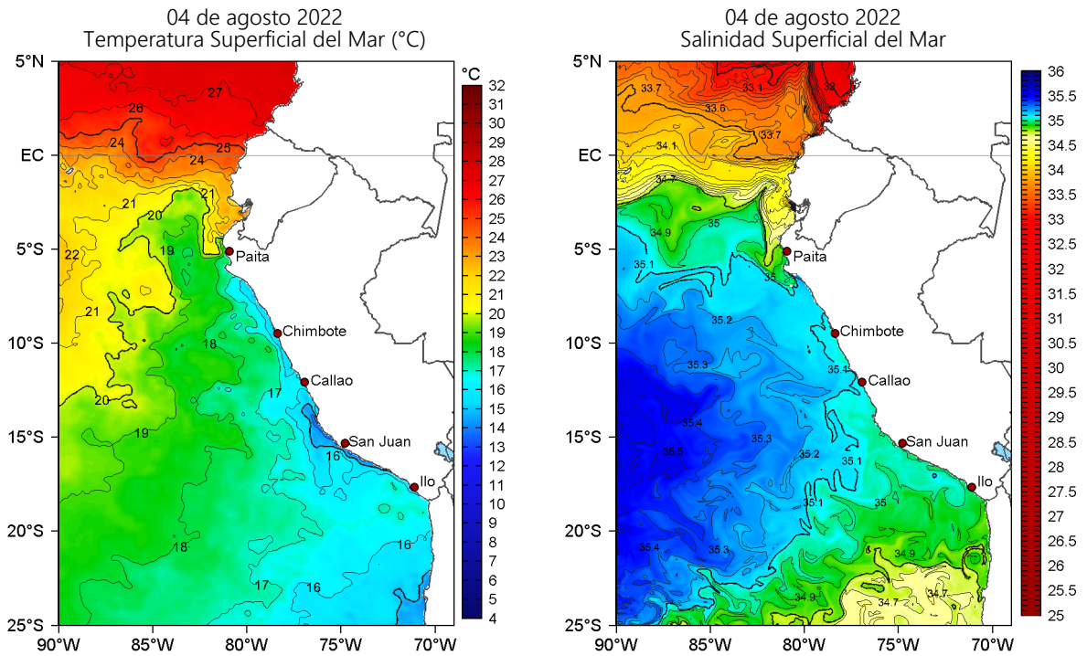
Figura 2. Temperatura superficial del mar (a la izquierda) y Salinidad superficial del mar (a la derecha) para el 04 de agosto de 2022. Datos: OSTIA-UKMO-L4-GLOB-v2.0 (UK Met Office, 2012; Donlon et al, 2012) y Hybrid Coordinate Ocean Model v. GOFS 3.1 (HYCOM; Halliwell et al., 1998; 2000; Bleck, 2001), respectivamente.
