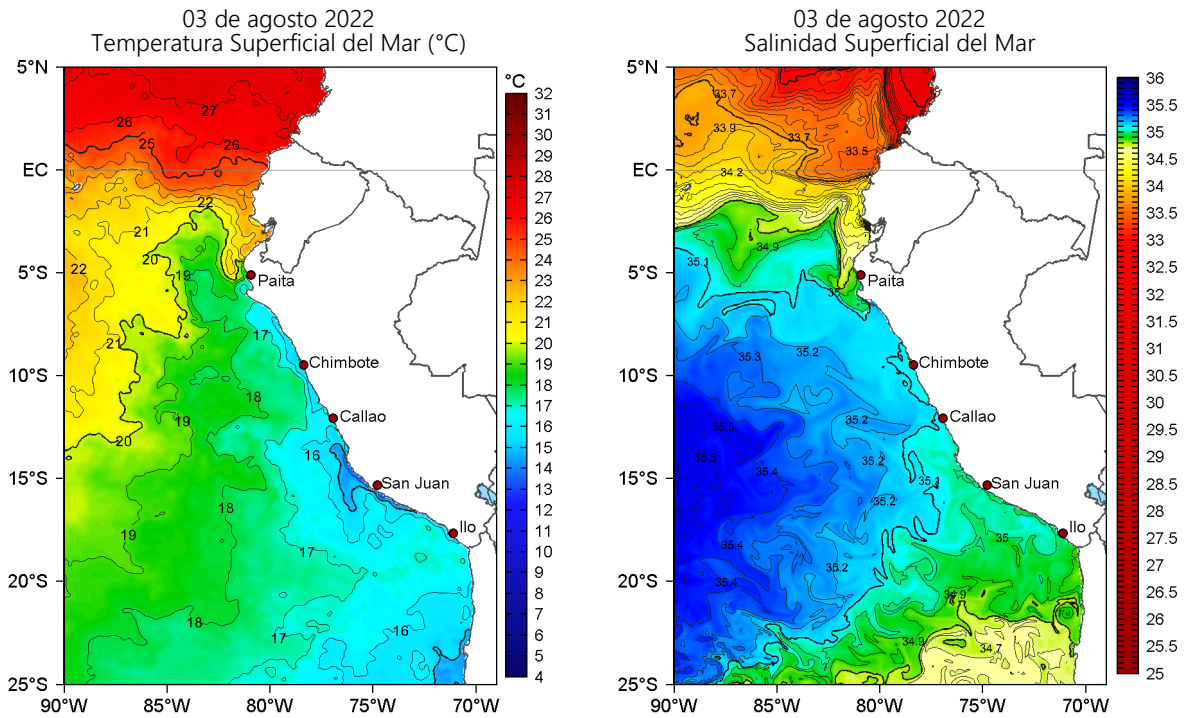
Figura 2. Temperatura superficial del mar (a la izquierda) y Salinidad superficial del mar (a la derecha) para el 03 de agosto de 2022. Datos: OSTIA-UKMO-L4-GLOB-v2.0 (UK Met Office, 2012; Donlon et al, 2012) y Hybrid Coordinate Ocean Model v. GOFS 3.1 (HYCOM; Halliwell et al., 1998; 2000; Bleck, 2001), respectivamente.
