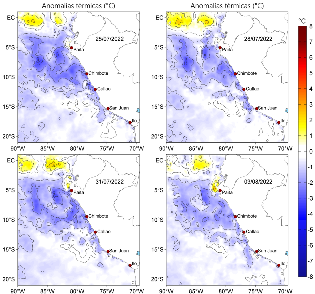
Figura 3. Anomalías de la temperatura superficial del mar (°C) para el 25, 28 y 31 de julio, así como para el 03 de agosto de 2022. Las anomalías se calcularon respecto de la climatología para el periodo 2007-2016. Datos: OSTIA-UKMO-L4-GLOB-v2.0 (UK Met Office, 2012; Donlon et al, 2012).
