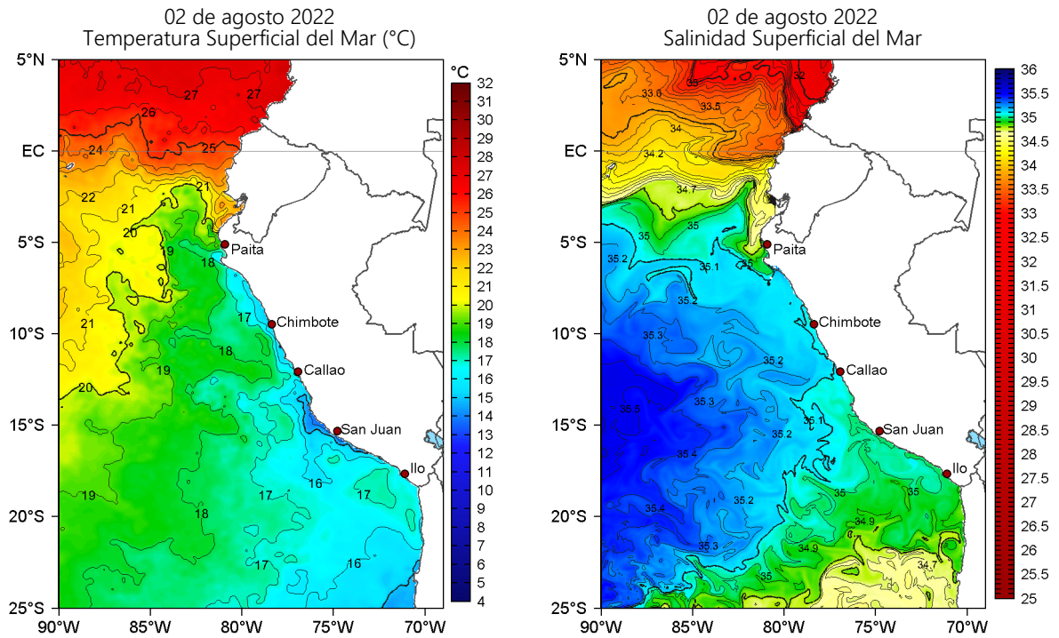
Figura 2. Temperatura superficial del mar (a la izquierda) y Salinidad superficial del mar (a la derecha) para el 02 de agosto de 2022. Datos: OSTIA-UKMO-L4-GLOB-v2.0 (UK Met Office, 2012; Donlon et al, 2012) y Hybrid Coordinate Ocean Model v. GOFS 3.1 (HYCOM; Halliwell et al., 1998; 2000; Bleck, 2001), respectivamente.
