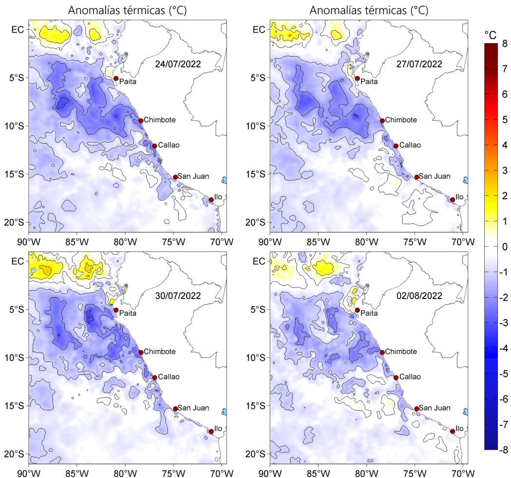
Figura 3. Anomalías de la temperatura superficial del mar (°C) para el 24, 27 y 30 de julio, así como para el 02 de agosto de 2022. Las anomalías se calcularon respecto de la climatología para el periodo 2007-2016. Datos: OSTIA-UKMO-L4-GLOB-v2.0 (UK Met Office, 2012; Donlon et al, 2012).
