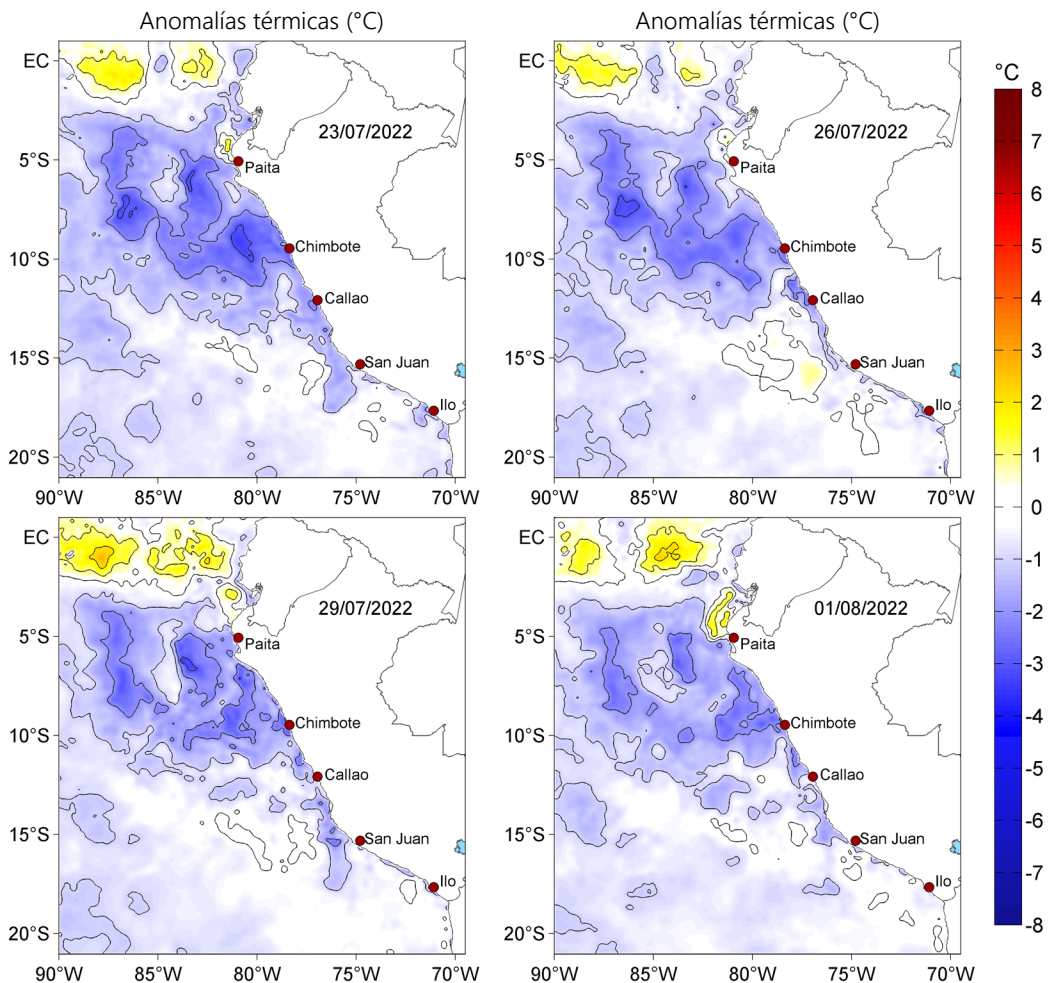
Figura 3. Anomalías de la temperatura superficial del mar (°C) para el 23, 26 y 29 de julio, así como para el 01 de agosto de 2022. Las anomalías se calcularon respecto de la climatología para el periodo 2007-2016. Datos: OSTIA-UKMO-L4-GLOB-v2.0 (UK Met Office, 2012; Donlon et al, 2012).
