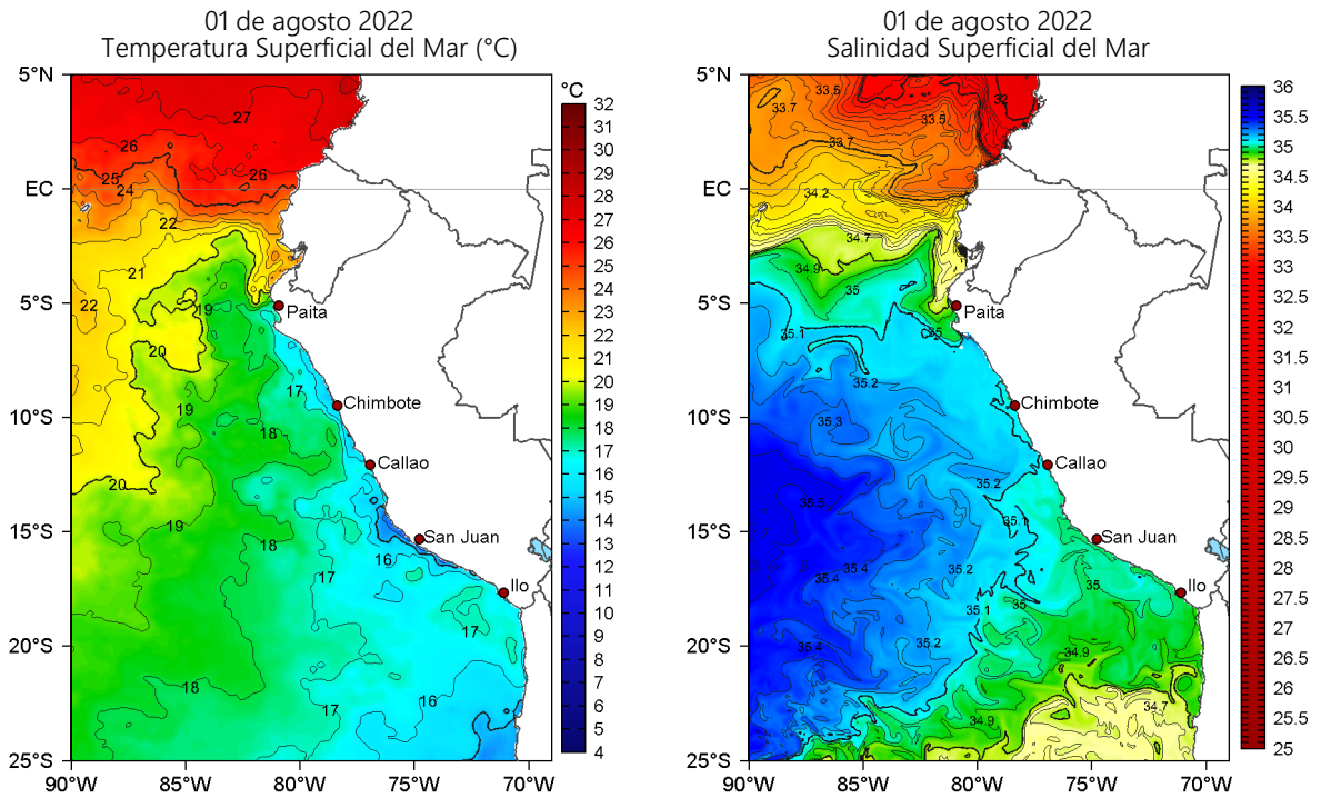
Figura 2. Temperatura superficial del mar (a la izquierda) y Salinidad superficial del mar (a la derecha) para el 01 de agosto de 2022. Datos: OSTIA-UKMO-L4-GLOB-v2.0 (UK Met Office, 2012; Donlon et al, 2012) y Hybrid Coordinate Ocean Model v. GOFS 3.1 (HYCOM; Halliwell et al., 1998; 2000; Bleck, 2001), respectivamente.
