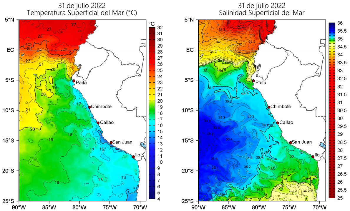
Figura 2. Temperatura superficial del mar (a la izquierda) y Salinidad superficial del mar (a la derecha) para el 31 de julio de 2022. Datos: OSTIA-UKMO-L4-GLOB-v2.0 (UK Met Office, 2012; Donlon et al, 2012) y Hybrid Coordinate Ocean Model v. GOFS 3.1 (HYCOM; Halliwell et al., 1998; 2000; Bleck, 2001), respectivamente.
