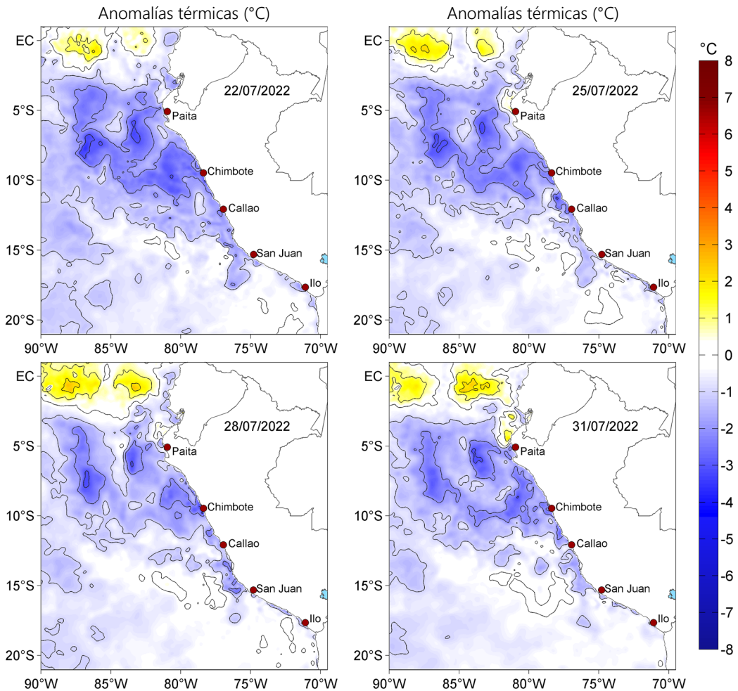
Figura 3. Anomalías de la temperatura superficial del mar (°C) para el 22, 25, 28 y 31 de julio de 2022. Las anomalías se calcularon respecto de la climatología para el periodo 2007-2016. Datos: OSTIA-UKMO-L4-GLOB-v2.0 (UK Met Office, 2012; Donlon et al, 2012).
