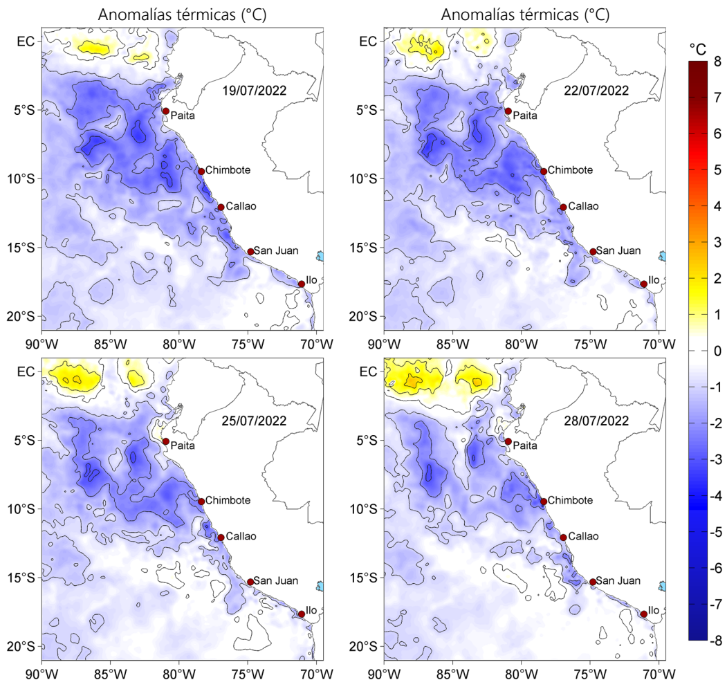
Figura 3. Anomalías de la temperatura superficial del mar (°C) para el 19, 22, 25 y 28 de julio de 2022. Las anomalías se calcularon respecto de la climatología para el periodo 2007-2016. Datos: OSTIA-UKMO-L4-GLOB-v2.0 (UK Met Office, 2012; Donlon et al, 2012).
