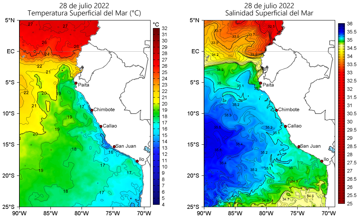
Figura 2. Temperatura superficial del mar (a la izquierda) y Salinidad superficial del mar (a la derecha) para el 28 de julio de 2022. Datos: OSTIA-UKMO-L4-GLOB-v2.0 (UK Met Office, 2012; Donlon et al, 2012) y Hybrid Coordinate Ocean Model v. GOFS 3.1 (HYCOM; Halliwell et al., 1998; 2000; Bleck, 2001), respectivamente.
