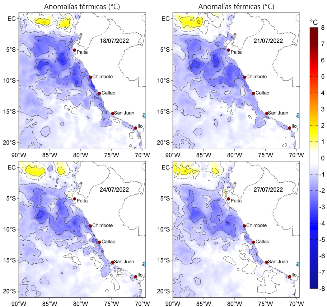
Figura 3. Anomalías de la temperatura superficial del mar (°C) para el 18, 21, 24 y 27 de julio de 2022. Las anomalías se calcularon respecto de la climatología para el periodo 2007-2016. Datos: OSTIA-UKMO-L4-GLOB-v2.0 (UK Met Office, 2012; Donlon et al, 2012).
