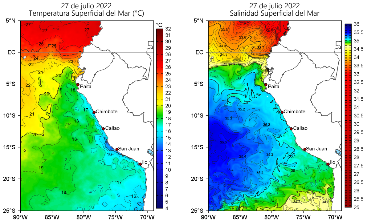
Figura 2. Temperatura superficial del mar (a la izquierda) y Salinidad superficial del mar (a la derecha) para el 27 de julio de 2022. Datos: OSTIA-UKMO-L4-GLOB-v2.0 (UK Met Office, 2012; Donlon et al, 2012) y Hybrid Coordinate Ocean Model v. GOFS 3.1 (HYCOM; Halliwell et al., 1998; 2000; Bleck, 2001), respectivamente.
