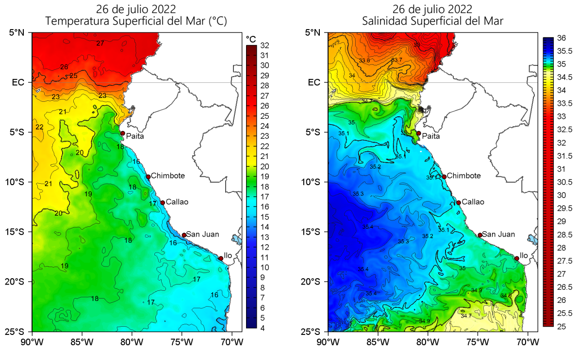
Figura 2. Temperatura superficial del mar (a la izquierda) y Salinidad superficial del mar (a la derecha) para el 26 de julio de 2022. Datos: OSTIA-UKMO-L4-GLOB-v2.0 (UK Met Office, 2012; Donlon et al, 2012) y Hybrid Coordinate Ocean Model v. GOFS 3.1 (HYCOM; Halliwell et al., 1998; 2000; Bleck, 2001), respectivamente.
