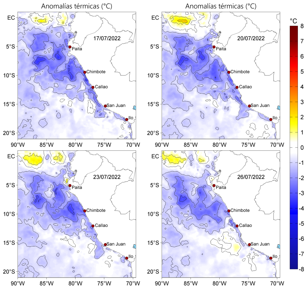
Figura 3. Anomalías de la temperatura superficial del mar (°C) para el 17, 20, 23 y 26 de julio de 2022. Las anomalías se calcularon respecto de la climatología para el periodo 2007-2016. Datos: OSTIA-UKMO-L4-GLOB-v2.0 (UK Met Office, 2012; Donlon et al, 2012).
