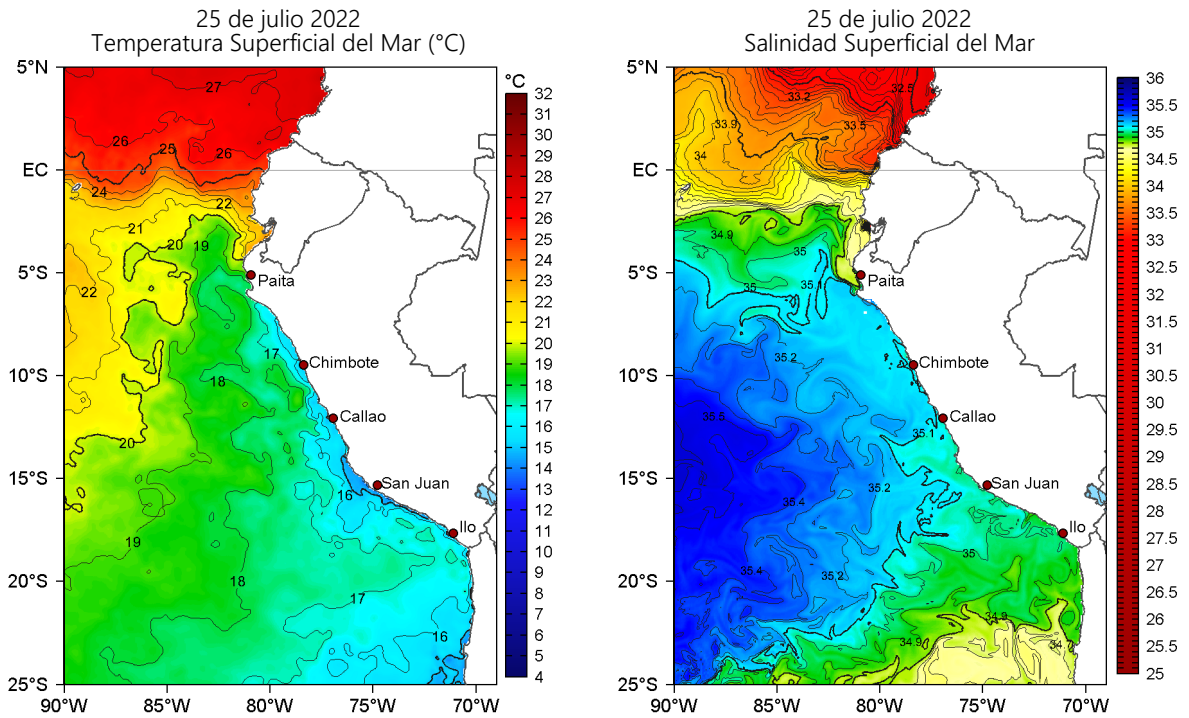
Figura 2. Temperatura superficial del mar (a la izquierda) y Salinidad superficial del mar (a la derecha) para el 25 de julio de 2022. Datos: OSTIA-UKMO-L4-GLOB-v2.0 (UK Met Office, 2012; Donlon et al, 2012) y Hybrid Coordinate Ocean Model v. GOFS 3.1 (HYCOM; Halliwell et al., 1998; 2000; Bleck, 2001), respectivamente.
