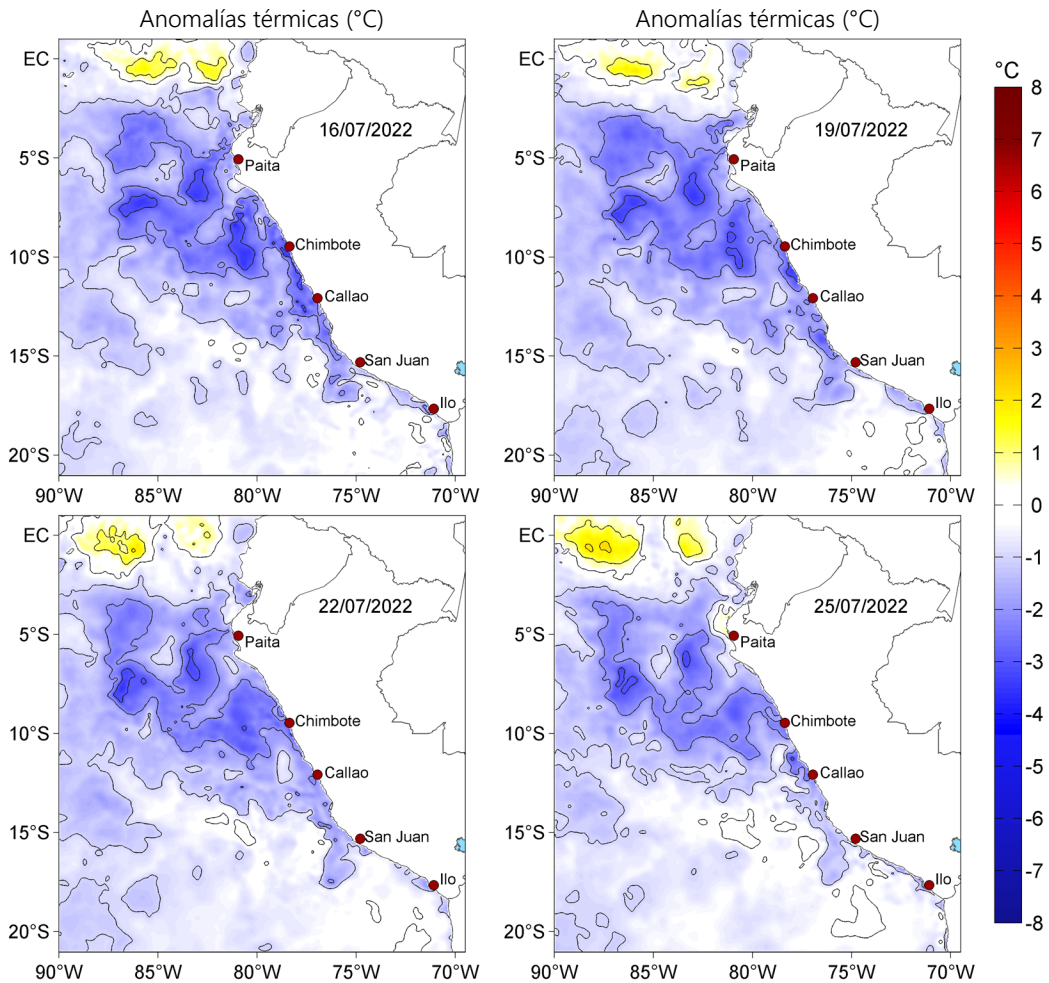
Figura 3. Anomalías de la temperatura superficial del mar (°C) para el 16, 19, 22 y 25 de julio de 2022. Las anomalías se calcularon respecto de la climatología para el periodo 2007-2016. Datos: OSTIA-UKMO-L4-GLOB-v2.0 (UK Met Office, 2012; Donlon et al, 2012).
