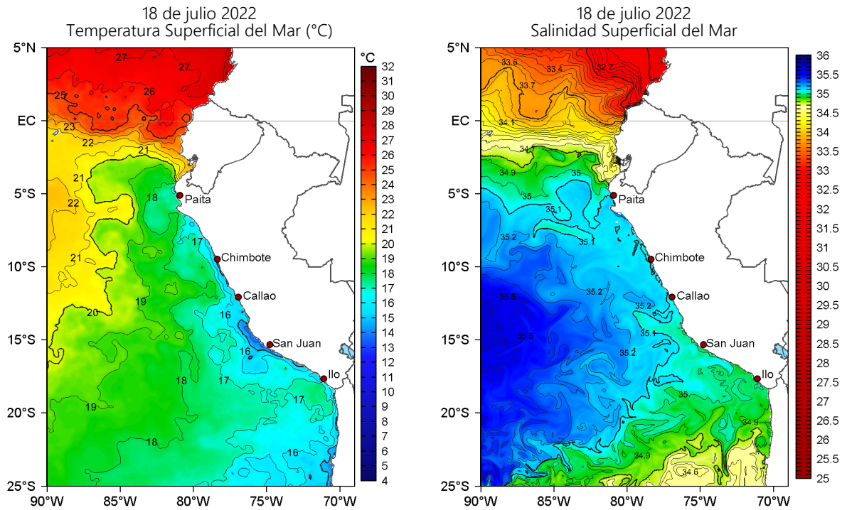
Figura 2. Temperatura superficial del mar (a la izquierda) y Salinidad superficial del mar (a la derecha) para el 18 de julio de 2022. Datos: OSTIA-UKMO-L4-GLOB-v2.0 (UK Met Office, 2012; Donlon et al, 2012) y Hybrid Coordinate Ocean Model v. GOFS 3.1 (HYCOM; Halliwell et al., 1998; 2000; Bleck, 2001), respectivamente.
