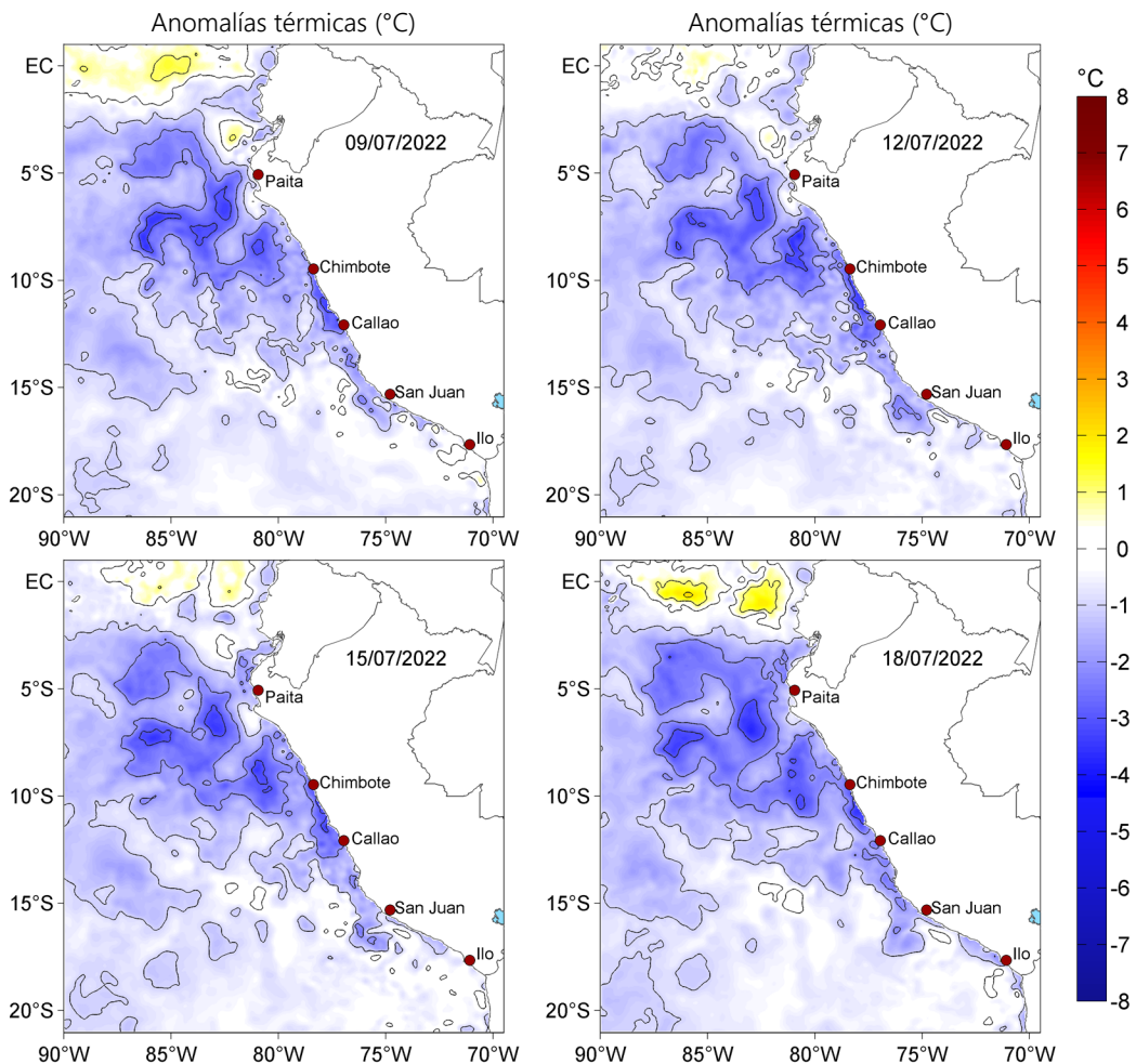
Figura 3. Anomalías de la temperatura superficial del mar (°C) para el 09, 12, 15 y 18 de julio de 2022. Las anomalías se calcularon respecto de la climatología para el periodo 2007-2016. Datos: OSTIA-UKMO-L4-GLOB-v2.0 (UK Met Office, 2012; Donlon et al, 2012).
