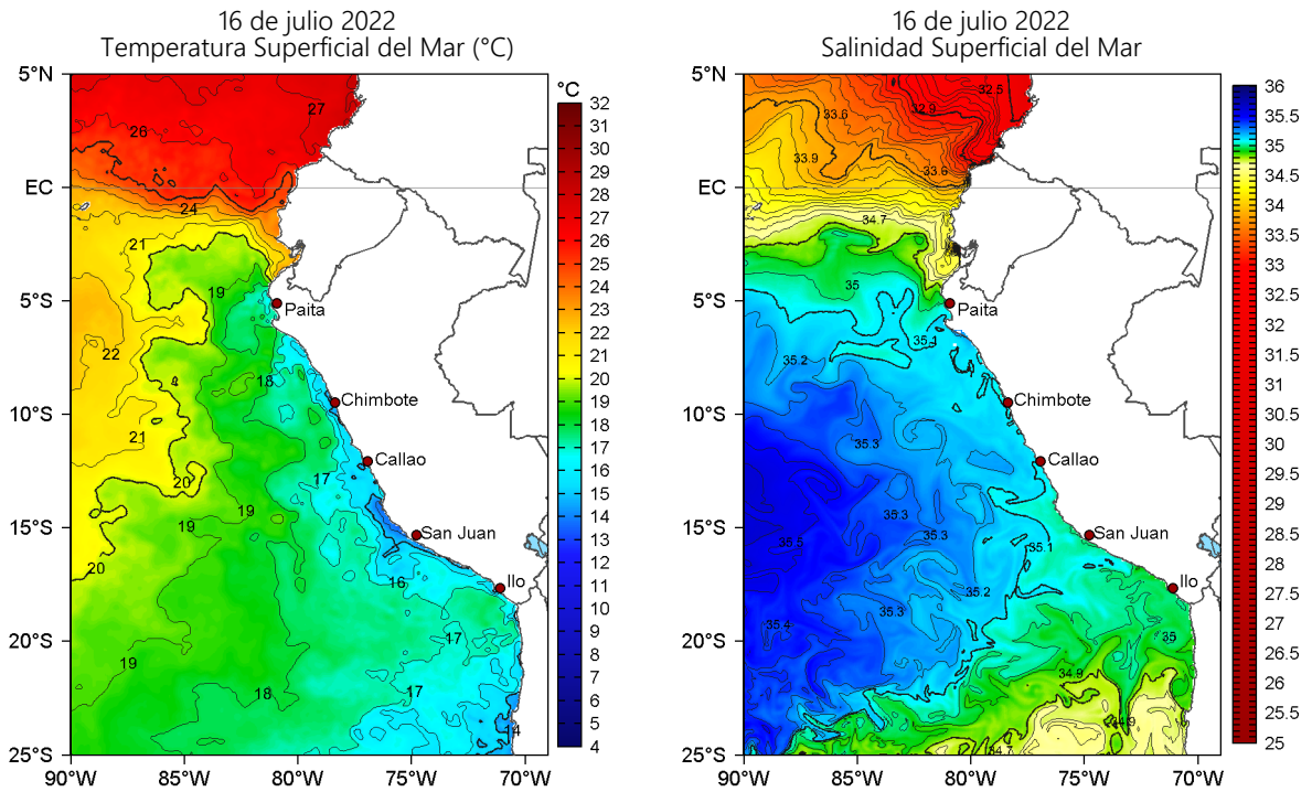
Figura 2. Temperatura superficial del mar (a la izquierda) y Salinidad superficial del mar (a la derecha) para el 16 de julio de 2022. Datos: OSTIA-UKMO-L4-GLOB-v2.0 (UK Met Office, 2012; Donlon et al, 2012) y Hybrid Coordinate Ocean Model v. GOFS 3.1 (HYCOM; Halliwell et al., 1998; 2000; Bleck, 2001), respectivamente.
