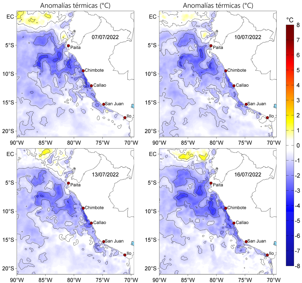
Figura 3. Anomalías de la temperatura superficial del mar (°C) para el 07, 10, 13 y 16 de julio de 2022. Las anomalías se calcularon respecto de la climatología para el periodo 2007-2016. Datos: OSTIA-UKMO-L4-GLOB-v2.0 (UK Met Office, 2012; Donlon et al, 2012).
