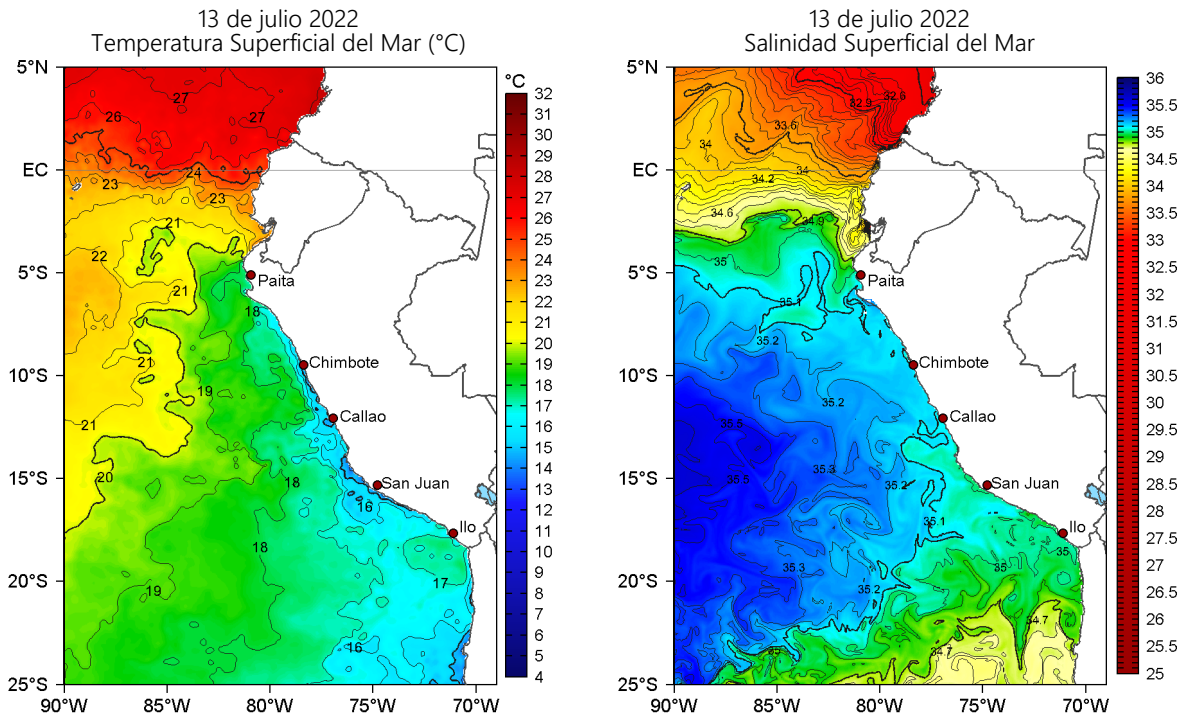
Figura 2. Temperatura superficial del mar (a la izquierda) y Salinidad superficial del mar (a la derecha) para el 13 de julio de 2022. Datos: OSTIA-UKMO-L4-GLOB-v2.0 (UK Met Office, 2012; Donlon et al, 2012) y Hybrid Coordinate Ocean Model v. GOFS 3.1 (HYCOM; Halliwell et al., 1998; 2000; Bleck, 2001), respectivamente.
