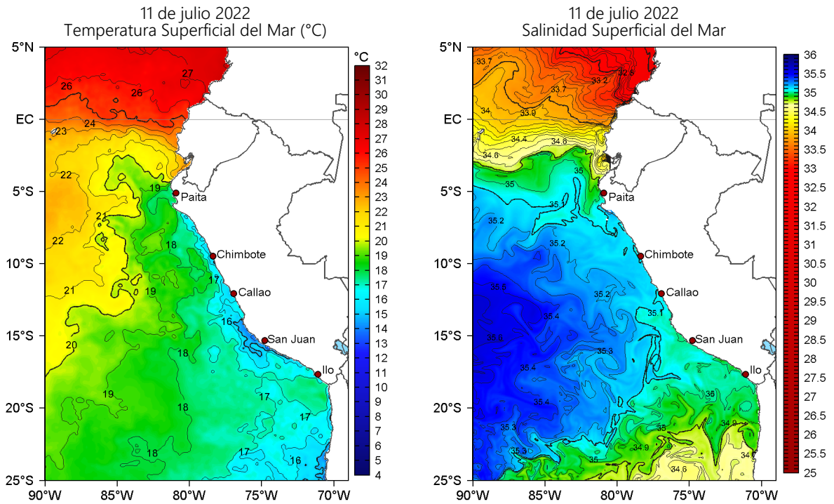
Figura 2. Temperatura superficial del mar (a la izquierda) y Salinidad superficial del mar (a la derecha) para el 11 de julio de 2022. Datos: OSTIA-UKMO-L4-GLOB-v2.0 (UK Met Office, 2012; Donlon et al, 2012) y Hybrid Coordinate Ocean Model v. GOFS 3.1 (HYCOM; Halliwell et al., 1998; 2000; Bleck, 2001), respectivamente.
