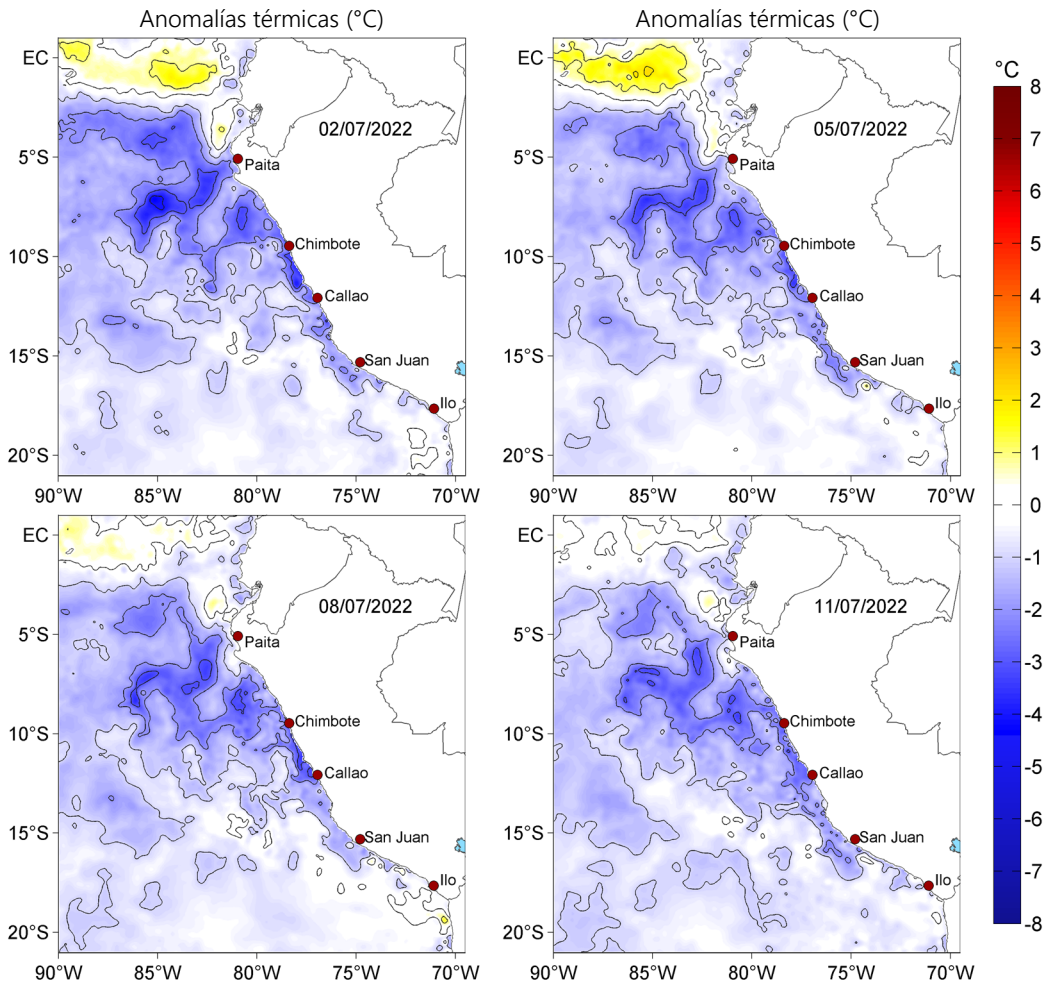
Figura 3. Anomalías de la temperatura superficial del mar (°C) para el 02, 05, 08 y 11 de julio de 2022. Las anomalías se calcularon respecto de la climatología para el periodo 2007-2016. Datos: OSTIA-UKMO-L4-GLOB-v2.0 (UK Met Office, 2012; Donlon et al, 2012).
