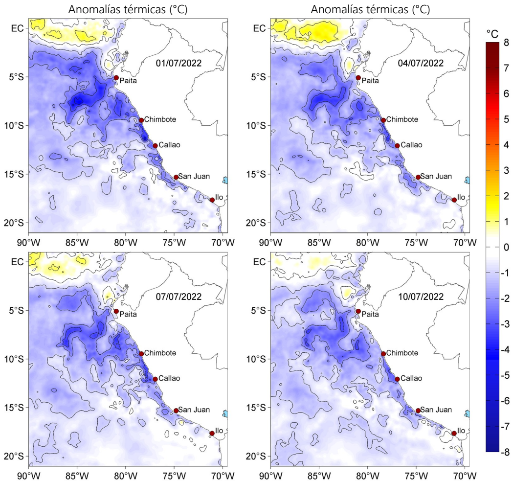
Figura 3. Anomalías de la temperatura superficial del mar (°C) para el 01, 04, 07 y 10 de julio de 2022. Las anomalías se calcularon respecto de la climatología para el periodo 2007-2016. Datos: OSTIA-UKMO-L4-GLOB-v2.0 (UK Met Office, 2012; Donlon et al, 2012).
