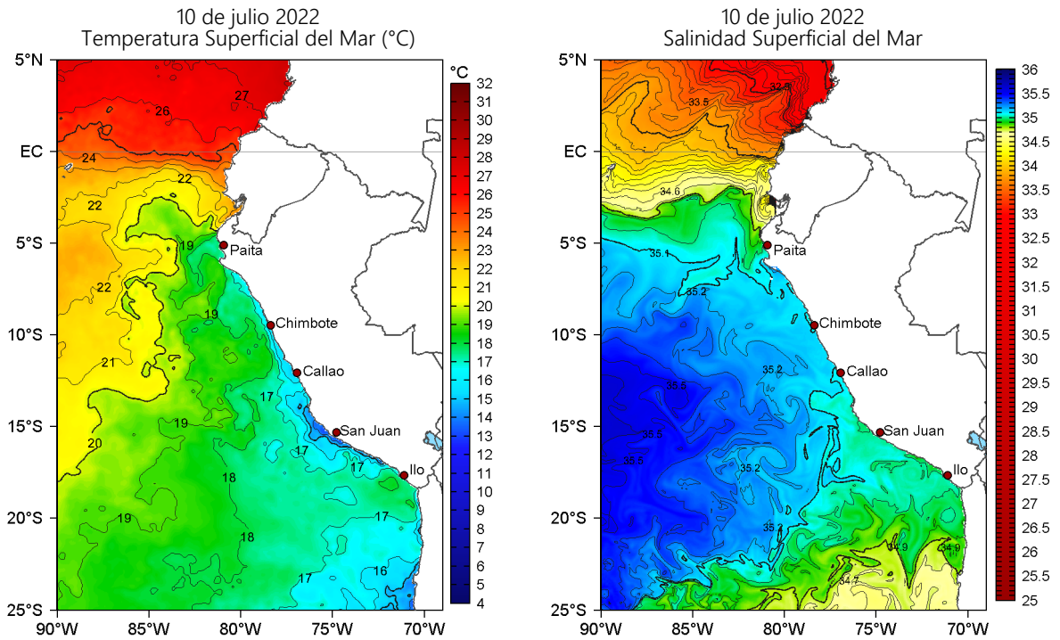
Figura 2. Temperatura superficial del mar (a la izquierda) y Salinidad superficial del mar (a la derecha) para el 10 de julio de 2022. Datos: OSTIA-UKMO-L4-GLOB-v2.0 (UK Met Office, 2012; Donlon et al, 2012) y Hybrid Coordinate Ocean Model v. GOFS 3.1 (HYCOM; Halliwell et al., 1998; 2000; Bleck, 2001), respectivamente.
