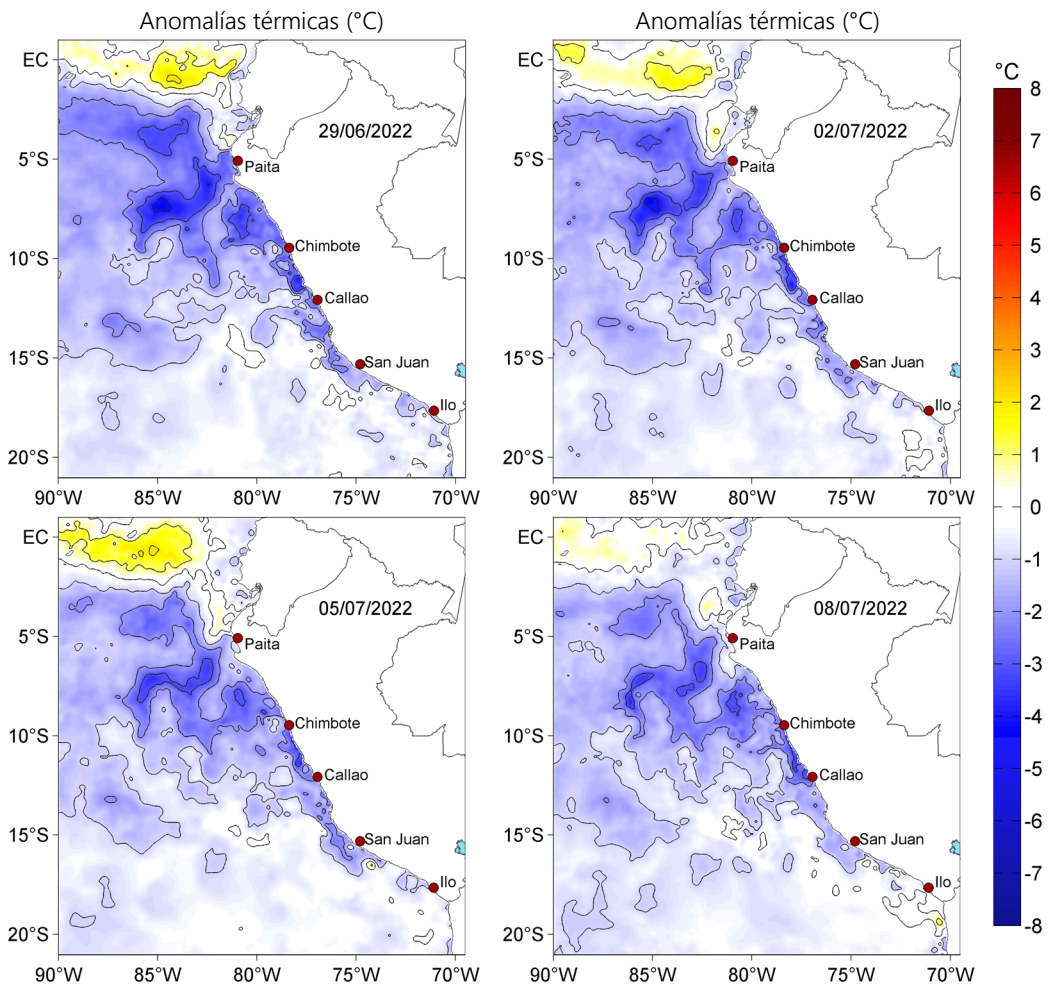
Figura 3. Anomalías de la temperatura superficial del mar (°C) para el 29 de junio, así como para el 02, 05 y 08 de julio de 2022. Las anomalías se calcularon respecto de la climatología para el periodo 2007-2016. Datos: OSTIA-UKMO-L4-GLOB-v2.0 (UK Met Office, 2012; Donlon et al, 2012).
