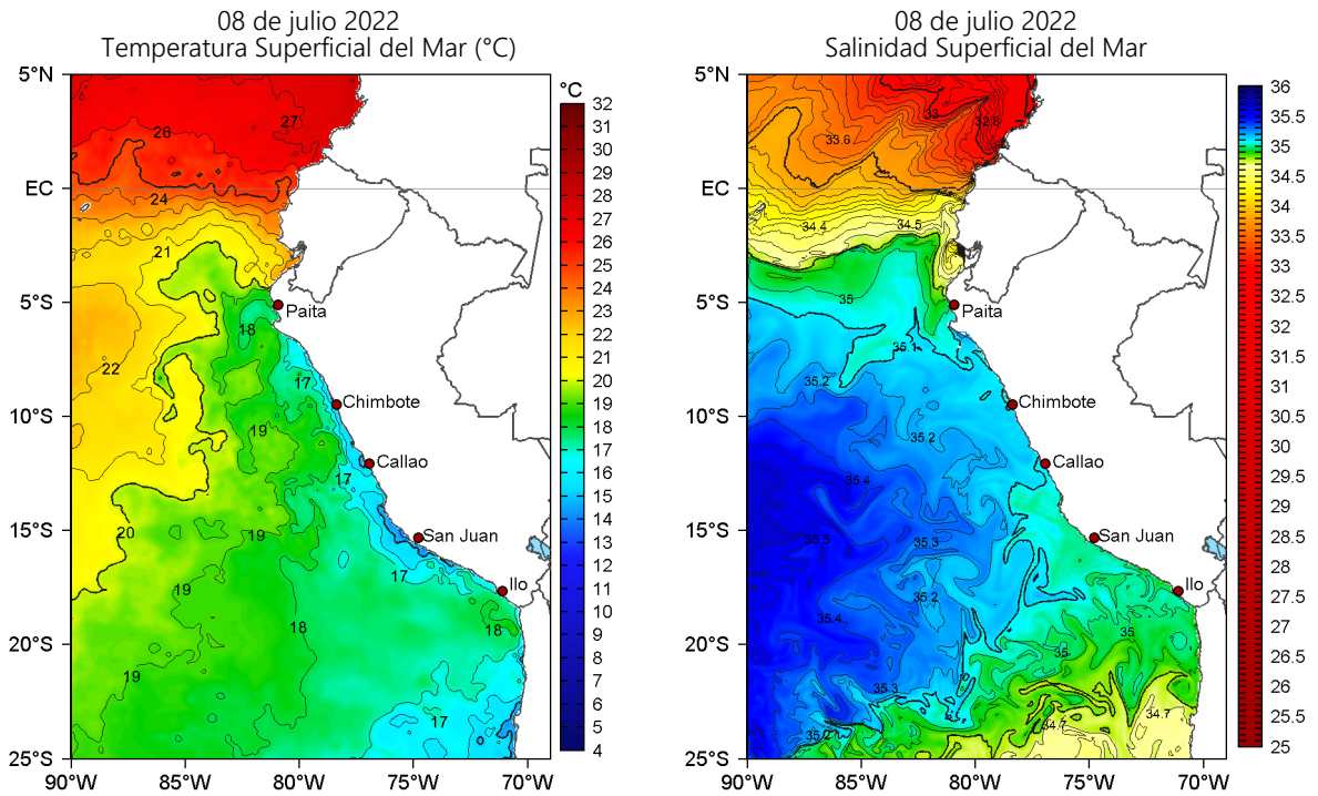
Figura 2. Temperatura superficial del mar (a la izquierda) y Salinidad superficial del mar (a la derecha) para el 08 de julio de 2022. Datos: OSTIA-UKMO-L4-GLOB-v2.0 (UK Met Office, 2012; Donlon et al, 2012) y Hybrid Coordinate Ocean Model v. GOFS 3.1 (HYCOM; Halliwell et al., 1998; 2000; Bleck, 2001), respectivamente.
