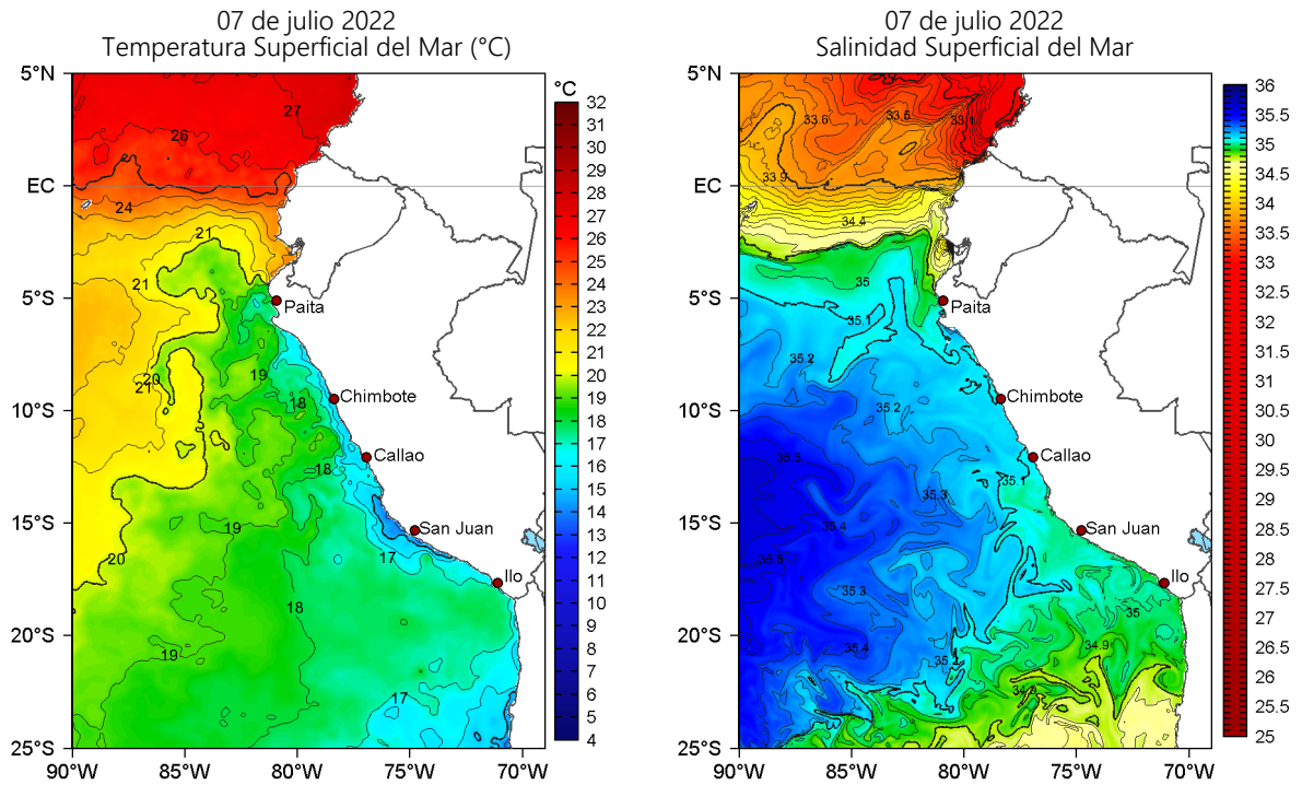
Figura 2. Temperatura superficial del mar (a la izquierda) y Salinidad superficial del mar (a la derecha) para el 07 de julio de 2022. Datos: OSTIA-UKMO-L4-GLOB-v2.0 (UK Met Office, 2012; Donlon et al, 2012) y Hybrid Coordinate Ocean Model v. GOFS 3.1 (HYCOM; Halliwell et al., 1998; 2000; Bleck, 2001), respectivamente.
