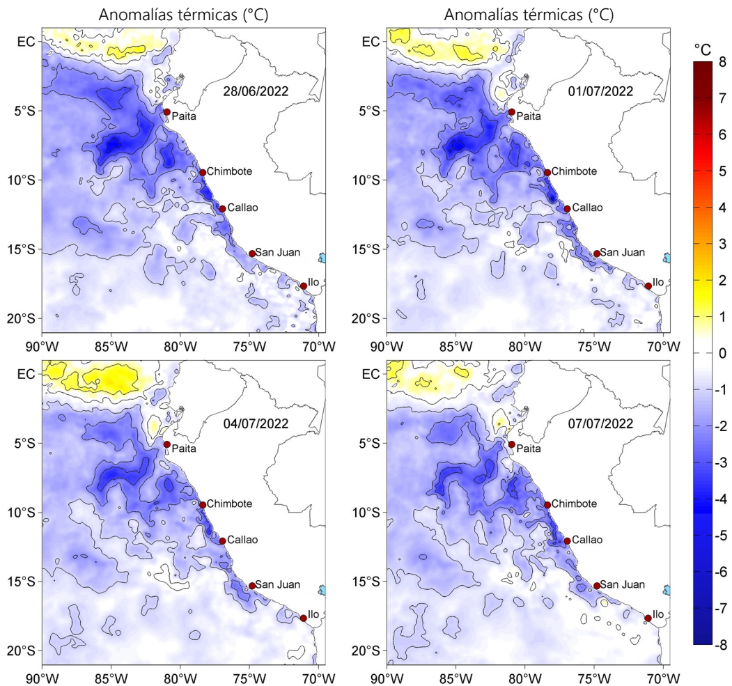
Figura 3. Anomalías de la temperatura superficial del mar (°C) para el 28 de junio, así como para el 01, 04 y 07 de julio de 2022. Las anomalías se calcularon respecto de la climatología para el periodo 2007-2016. Datos: OSTIA-UKMO-L4-GLOB-v2.0 (UK Met Office, 2012; Donlon et al, 2012).
