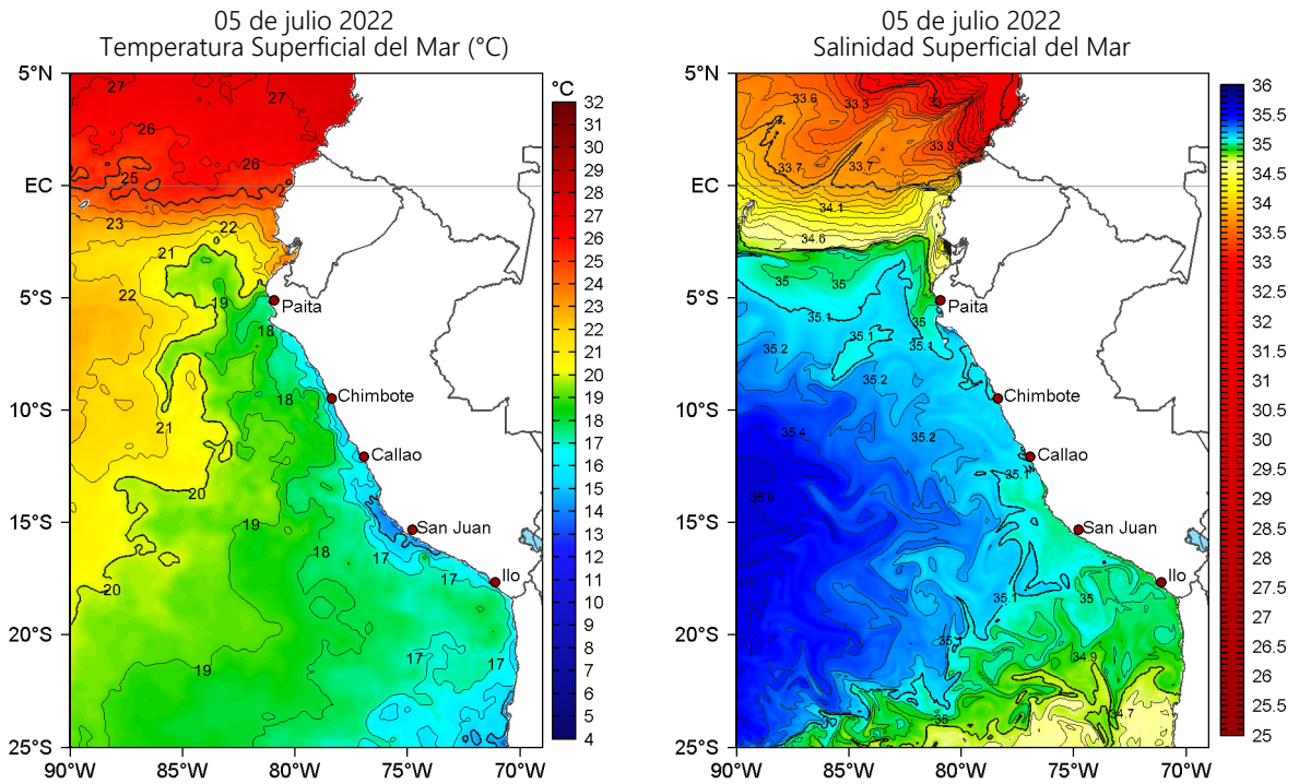
Figura 2. Temperatura superficial del mar (a la izquierda) y Salinidad superficial del mar (a la derecha) para el 05 de julio de 2022. Datos: OSTIA-UKMO-L4-GLOB-v2.0 (UK Met Office, 2012; Donlon et al, 2012) y Hybrid Coordinate Ocean Model v. GOFS 3.1 (HYCOM; Halliwell et al., 1998; 2000; Bleck, 2001), respectivamente.
