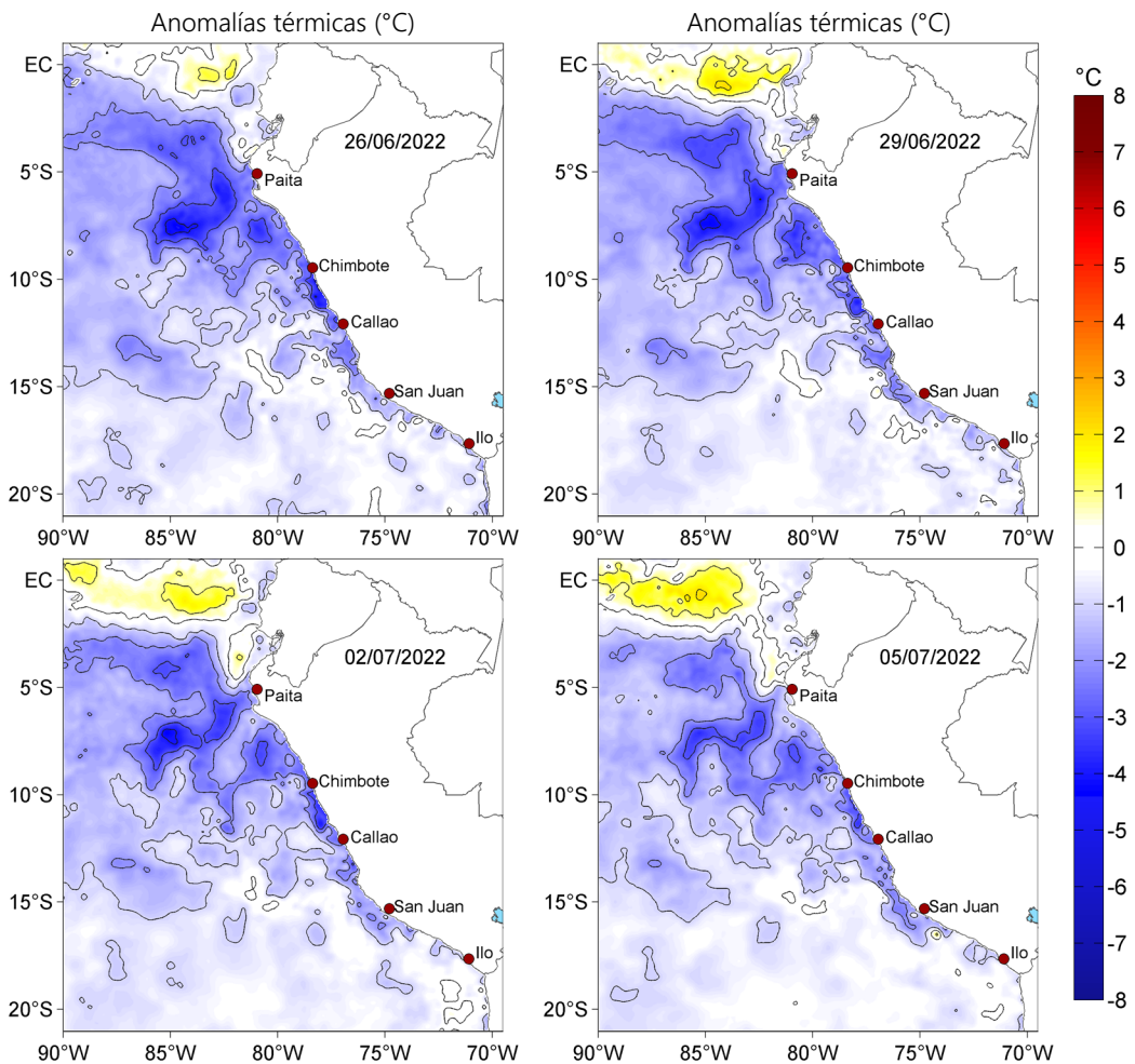
Figura 3. Anomalías de la temperatura superficial del mar (°C) para el 26 y 29 de junio, así como para el 02 y 05 de julio de 2022. Las anomalías se calcularon respecto de la climatología para el periodo 2007-2016. Datos: OSTIA-UKMO-L4-GLOB-v2.0 (UK Met Office, 2012; Donlon et al, 2012).
