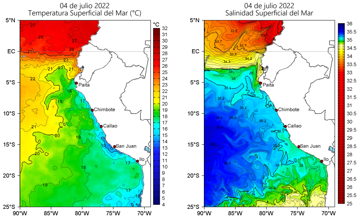
Figura 2. Temperatura superficial del mar (a la izquierda) y Salinidad superficial del mar (a la derecha) para el 04 de julio de 2022. Datos: OSTIA-UKMO-L4-GLOB-v2.0 (UK Met Office, 2012; Donlon et al, 2012) y Hybrid Coordinate Ocean Model v. GOFS 3.1 (HYCOM; Halliwell et al., 1998; 2000; Bleck, 2001), respectivamente.
