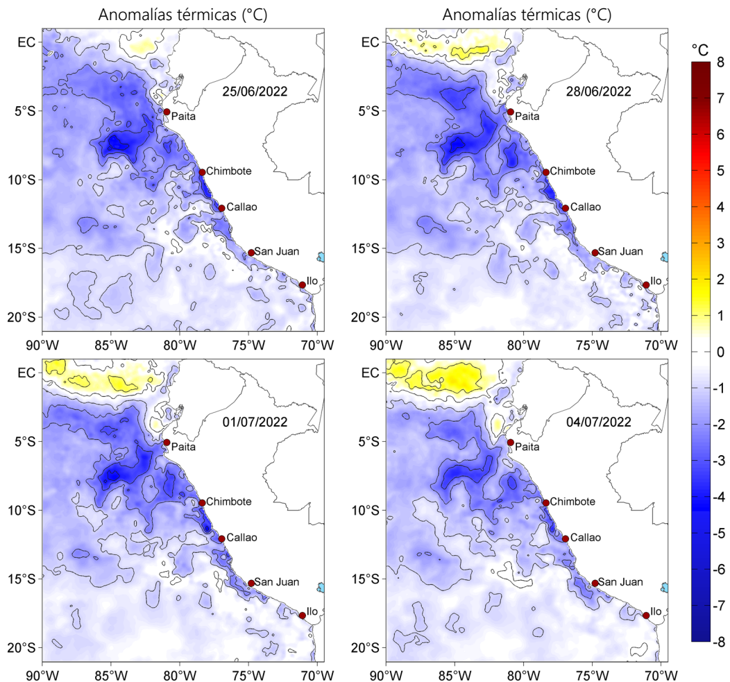
Figura 3. Anomalías de la temperatura superficial del mar (°C) para el 25 y 28 de junio, así como para el 01 y 04 de julio de 2022. Las anomalías se calcularon respecto de la climatología para el periodo 2007-2016. Datos: OSTIA-UKMO-L4-GLOB-v2.0 (UK Met Office, 2012; Donlon et al, 2012).
