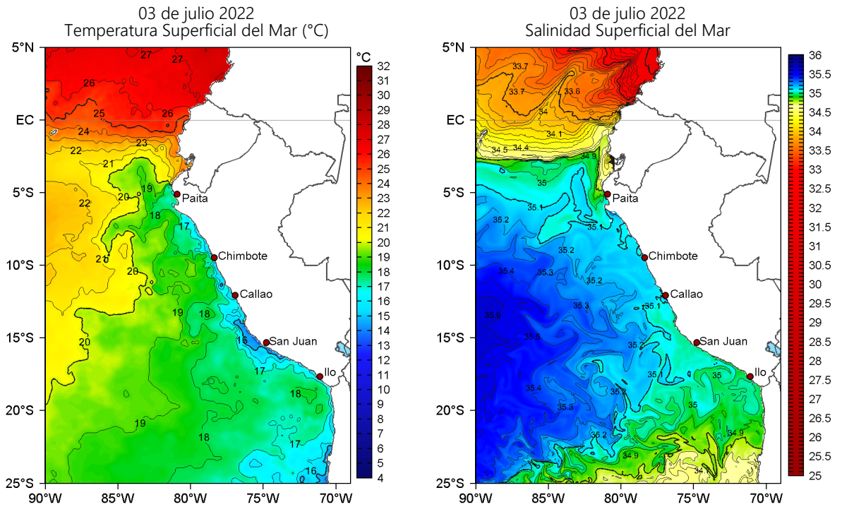
Figura 2. Temperatura superficial del mar (a la izquierda) y Salinidad superficial del mar (a la derecha) para el 03 de julio de 2022. Datos: OSTIA-UKMO-L4-GLOB-v2.0 (UK Met Office, 2012; Donlon et al, 2012) y Hybrid Coordinate Ocean Model v. GOFS 3.1 (HYCOM; Halliwell et al., 1998; 2000; Bleck, 2001), respectivamente.
