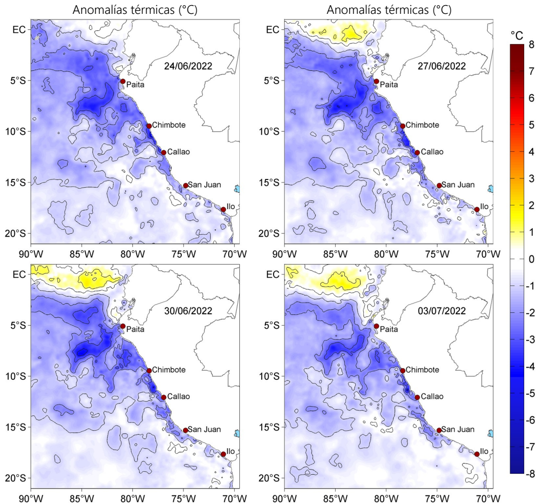
Figura 3. Anomalías de la temperatura superficial del mar (°C) para el 24, 27 y 30 de junio, así como para el 03 de julio de 2022. Las anomalías se calcularon respecto de la climatología para el periodo 2007-2016. Datos: OSTIA-UKMO-L4-GLOB-v2.0 (UK Met Office, 2012; Donlon et al, 2012).
