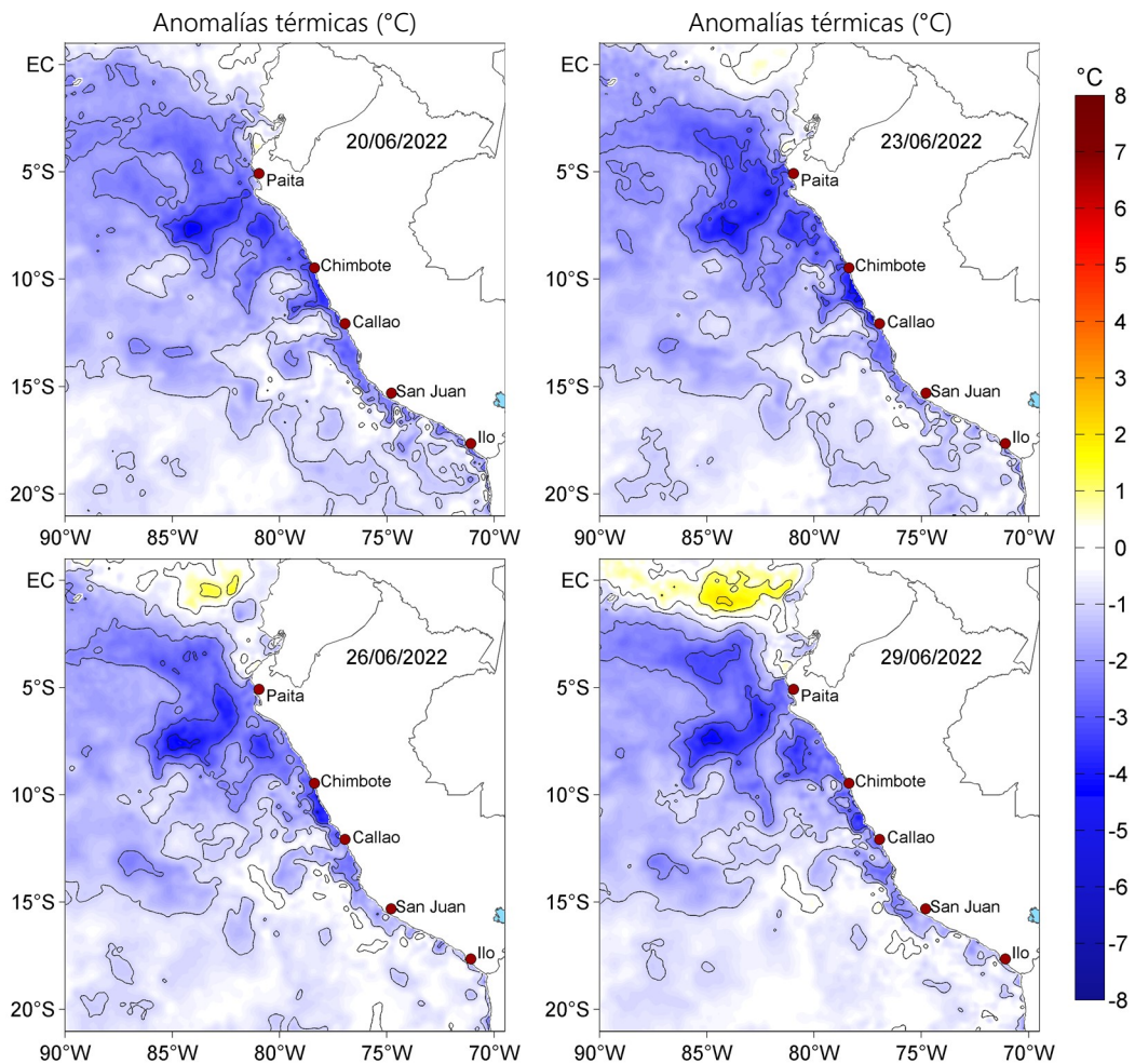
Figura 3. Anomalías de la temperatura superficial del mar (°C) para el 20, 23, 26 y 29 de junio de 2022. Las anomalías se calcularon respecto de la climatología para el periodo 2007-2016. Datos: OSTIA-UKMO-L4-GLOB-v2.0 (UK Met Office, 2012; Donlon et al, 2012).
