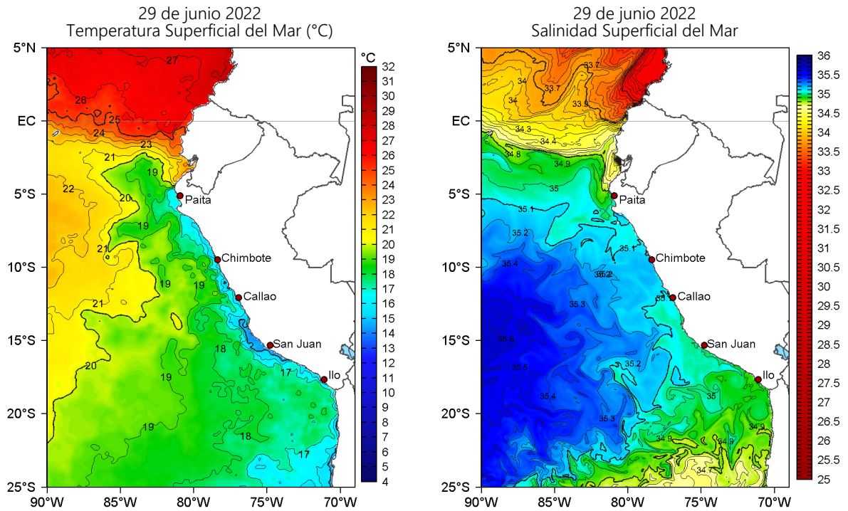
Figura 2. Temperatura superficial del mar (a la izquierda) y Salinidad superficial del mar (a la derecha) para el 29 de junio de 2022. Datos: OSTIA-UKMO-L4-GLOB-v2.0 (UK Met Office, 2012; Donlon et al, 2012) y Hybrid Coordinate Ocean Model v. GOFS 3.1 (HYCOM; Halliwell et al., 1998; 2000; Bleck, 2001), respectivamente.
