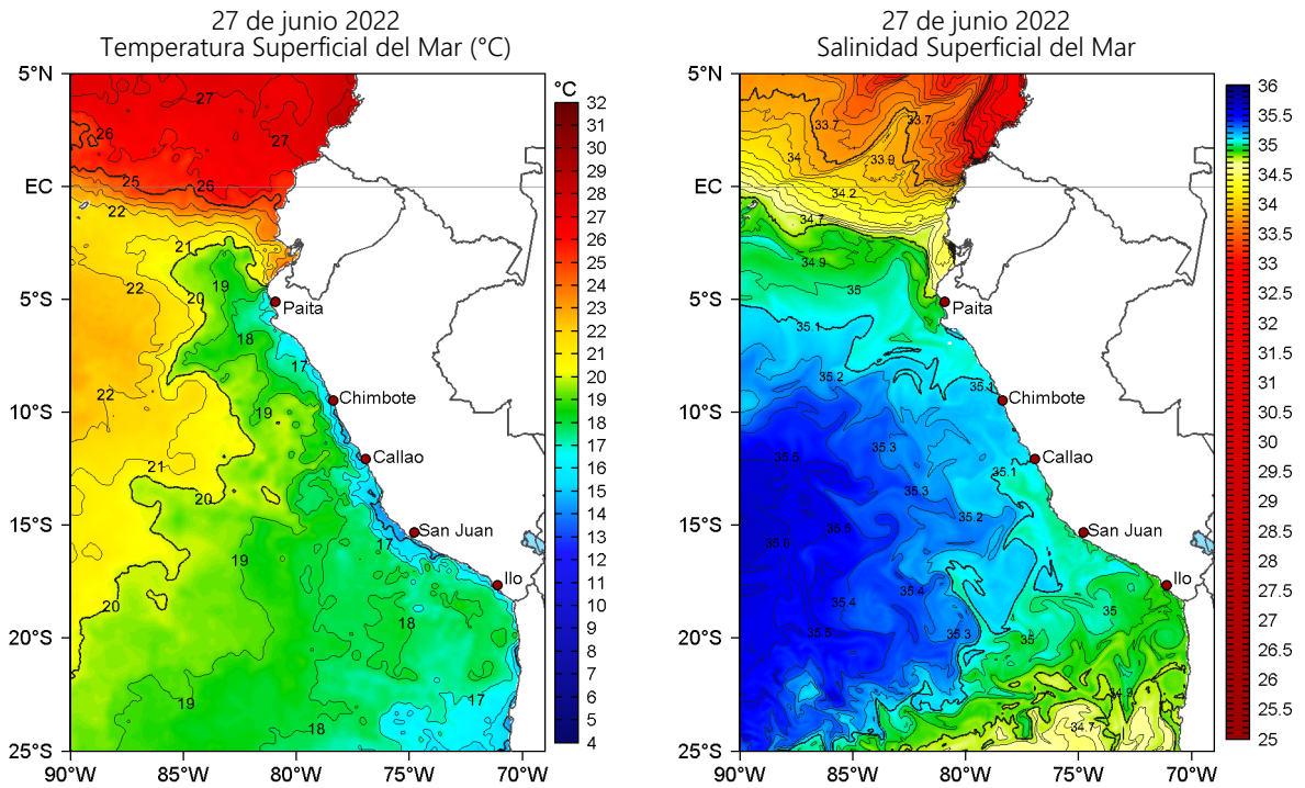
Figura 2. Temperatura superficial del mar (a la izquierda) y Salinidad superficial del mar (a la derecha) para el 27 de junio de 2022. Datos: OSTIA-UKMO-L4-GLOB-v2.0 (UK Met Office, 2012; Donlon et al, 2012) y Hybrid Coordinate Ocean Model v. GOFS 3.1 (HYCOM; Halliwell et al., 1998; 2000; Bleck, 2001), respectivamente.
