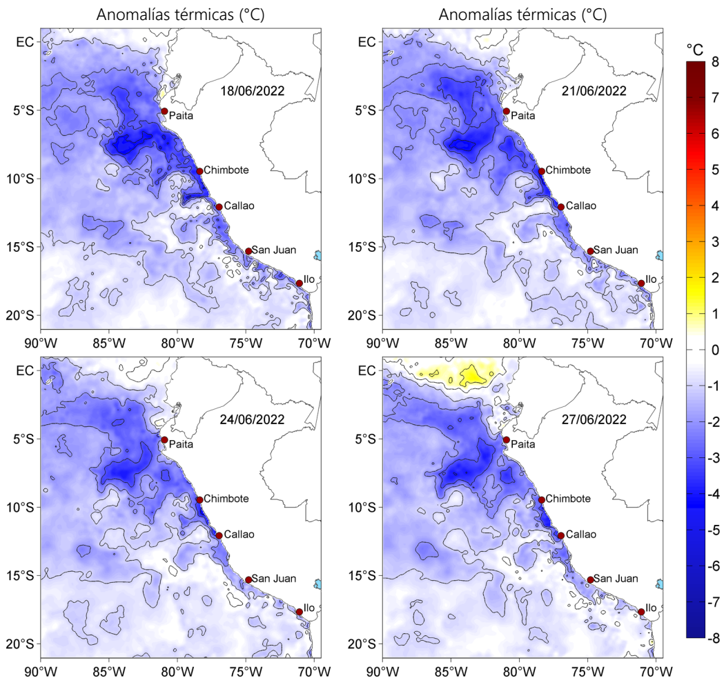
Figura 3. Anomalías de la temperatura superficial del mar (°C) para el 18, 21, 24 y 27 de junio de 2022. Las anomalías se calcularon respecto de la climatología para el periodo 2007-2016. Datos: OSTIA-UKMO-L4-GLOB-v2.0 (UK Met Office, 2012; Donlon et al, 2012).
