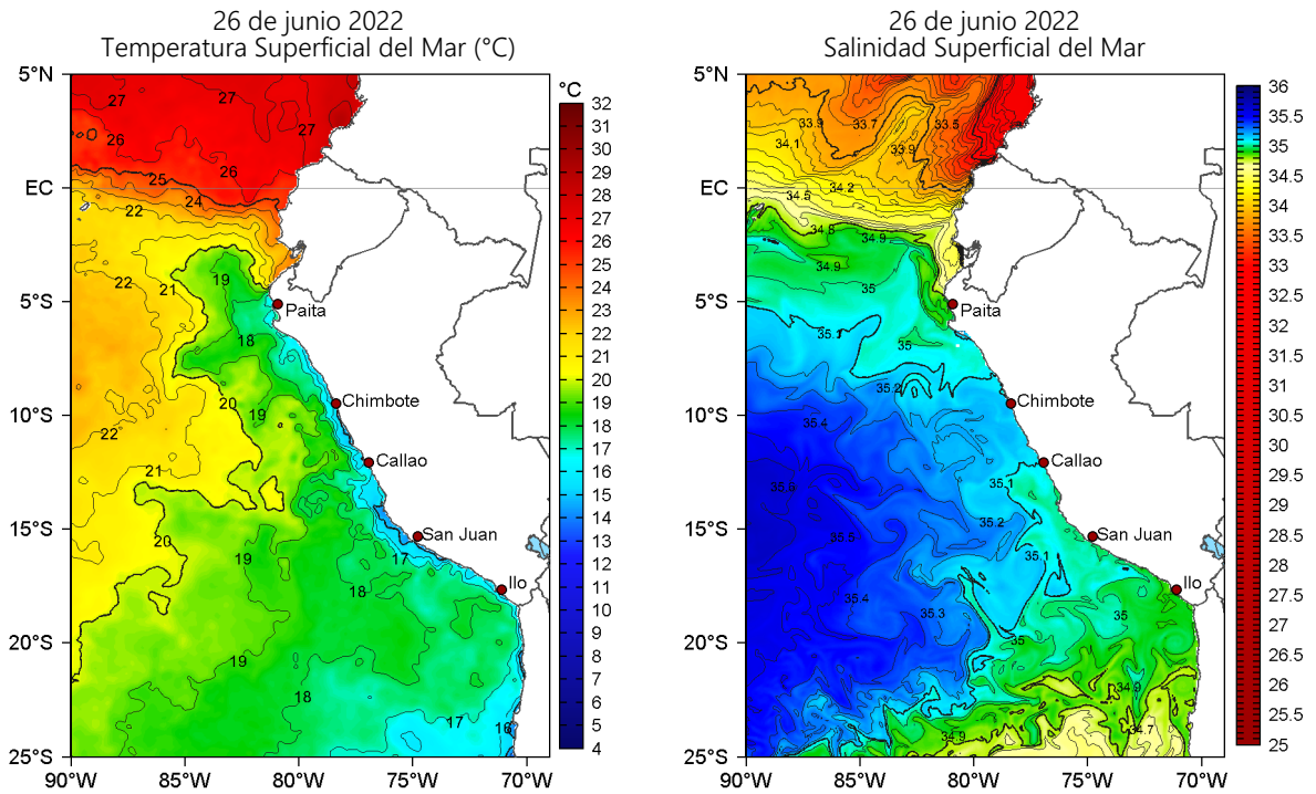
Figura 2. Temperatura superficial del mar (a la izquierda) y Salinidad superficial del mar (a la derecha) para el 26 de junio de 2022. Datos: OSTIA-UKMO-L4-GLOB-v2.0 (UK Met Office, 2012; Donlon et al, 2012) y Hybrid Coordinate Ocean Model v. GOFS 3.1 (HYCOM; Halliwell et al., 1998; 2000; Bleck, 2001), respectivamente.
