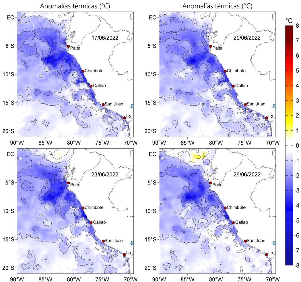
Figura 3. Anomalías de la temperatura superficial del mar (°C) para el 17, 20, 23 y 26 de junio de 2022. Las anomalías se calcularon respecto de la climatología para el periodo 2007-2016. Datos: OSTIA-UKMO-L4-GLOB-v2.0 (UK Met Office, 2012; Donlon et al, 2012).
