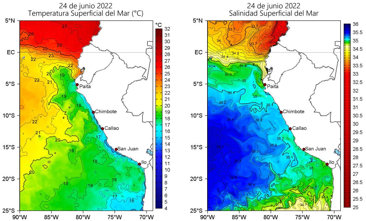
Figura 2. Temperatura superficial del mar (a la izquierda) y Salinidad superficial del mar (a la derecha) para el 24 de junio de 2022. Datos: OSTIA-UKMO-L4-GLOB-v2.0 (UK Met Office, 2012; Donlon et al, 2012) y Hybrid Coordinate Ocean Model v. GOFS 3.1 (HYCOM; Halliwell et al., 1998; 2000; Bleck, 2001), respectivamente.
