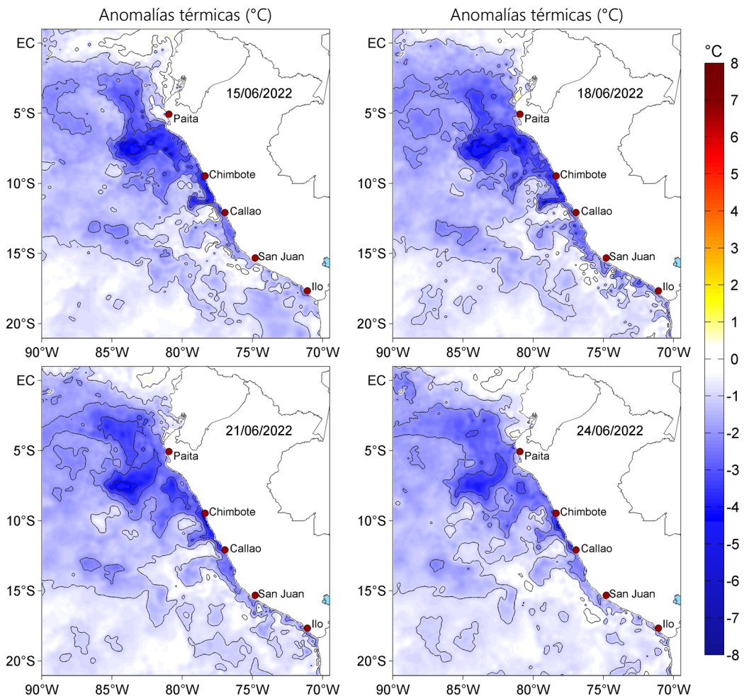
Figura 3. Anomalías de la temperatura superficial del mar (°C) para el 15, 18, 21 y 24 de junio de 2022. Las anomalías se calcularon respecto de la climatología para el periodo 2007-2016. Datos: OSTIA-UKMO-L4-GLOB-v2.0 (UK Met Office, 2012; Donlon et al, 2012).
