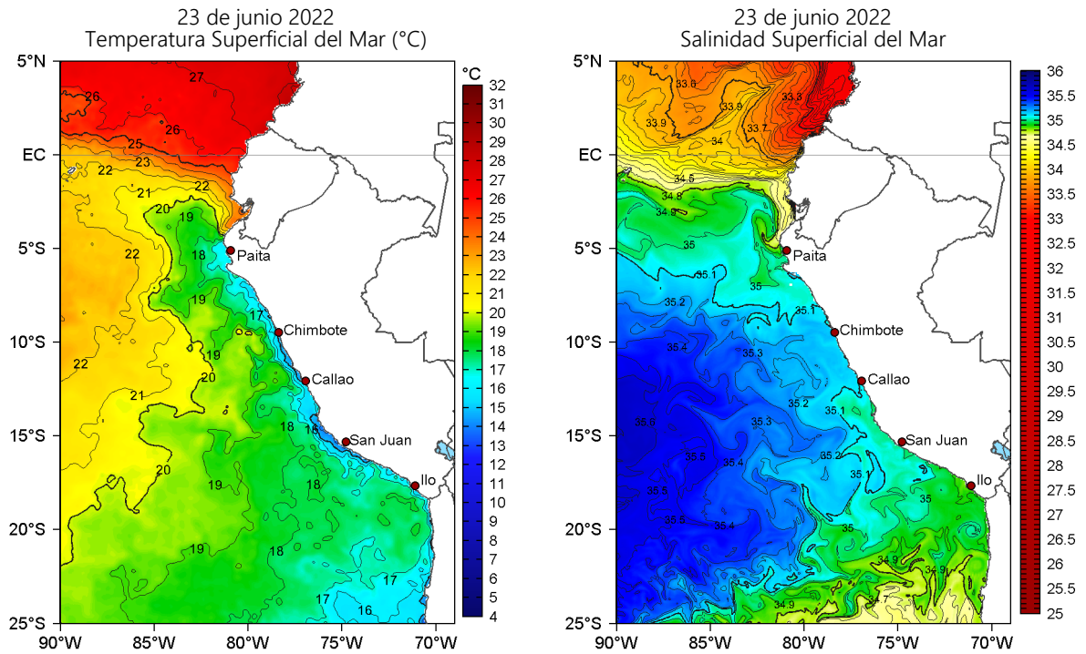
Figura 2. Temperatura superficial del mar (a la izquierda) y Salinidad superficial del mar (a la derecha) para el 23 de junio de 2022. Datos: OSTIA-UKMO-L4-GLOB-v2.0 (UK Met Office, 2012; Donlon et al, 2012) y Hybrid Coordinate Ocean Model v. GOFS 3.1 (HYCOM; Halliwell et al., 1998; 2000; Bleck, 2001), respectivamente.
