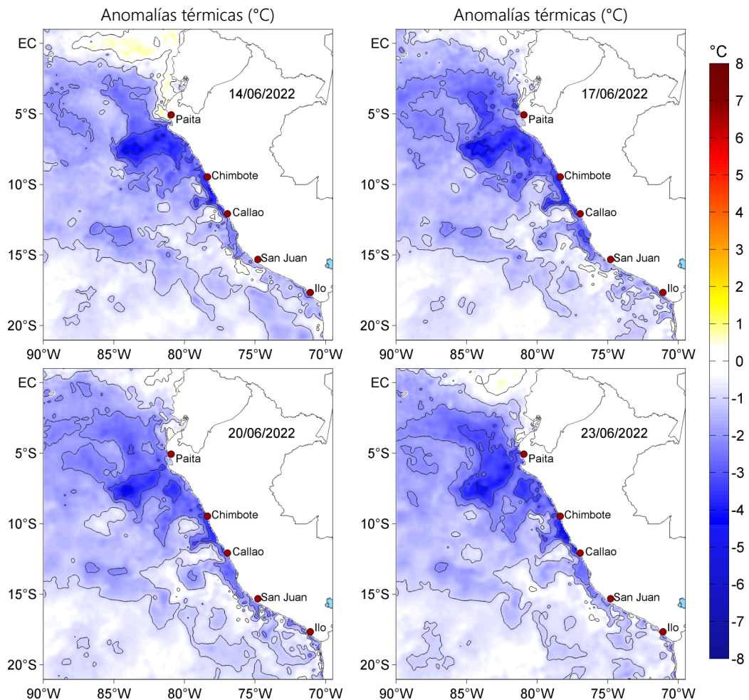
Figura 3. Anomalías de la temperatura superficial del mar (°C) para el 14, 17, 20 y 23 de junio de 2022. Las anomalías se calcularon respecto de la climatología para el periodo 2007-2016. Datos: OSTIA-UKMO-L4-GLOB-v2.0 (UK Met Office, 2012; Donlon et al, 2012).
