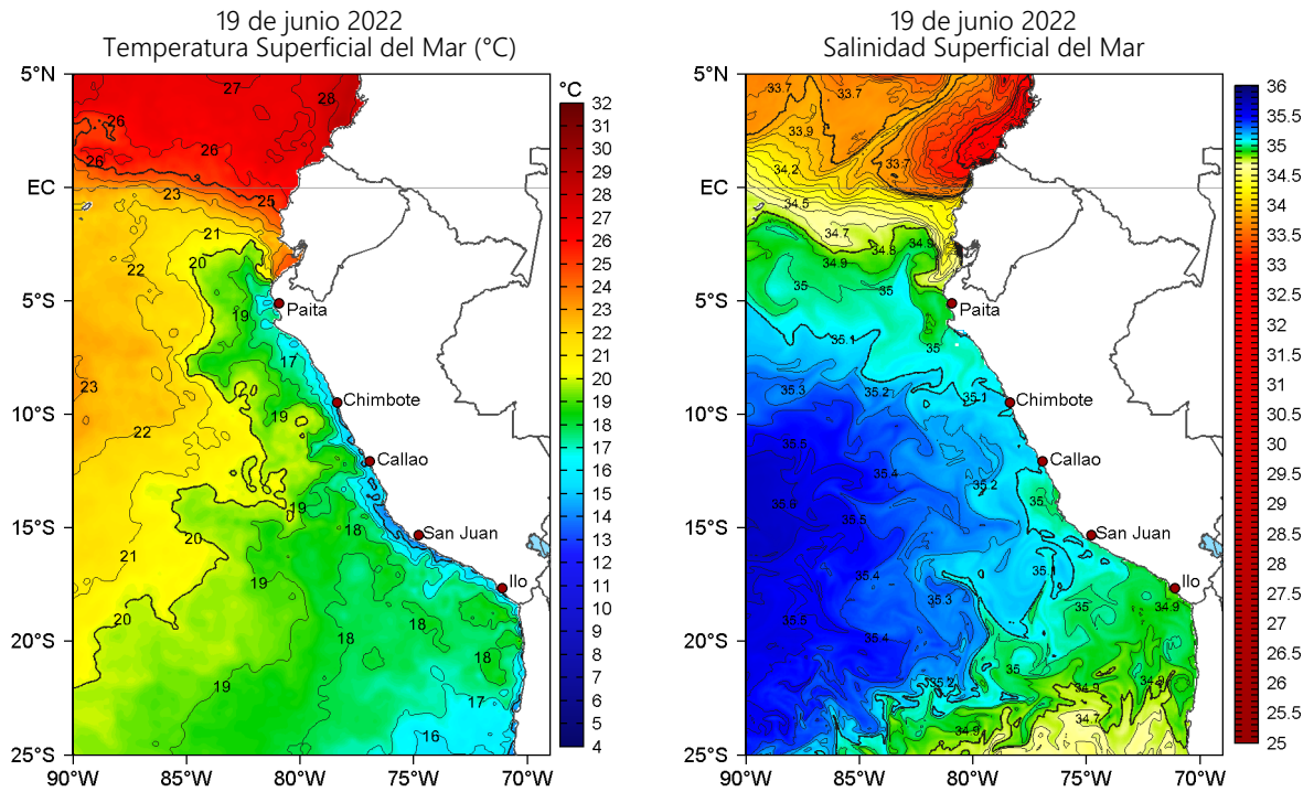
Figura 2. Temperatura superficial del mar (a la izquierda) y Salinidad superficial del mar (a la derecha) para el 19 de junio de 2022. Datos: OSTIA-UKMO-L4-GLOB-v2.0 (UK Met Office, 2012; Donlon et al, 2012) y Hybrid Coordinate Ocean Model v. GOFS 3.1 (HYCOM; Halliwell et al., 1998; 2000; Bleck, 2001), respectivamente.
