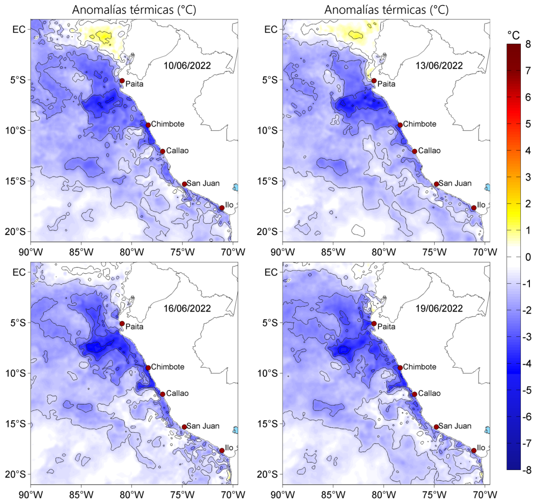
Figura 3. Anomalías de la temperatura superficial del mar (°C) para el 10, 13, 16 y 19 de junio de 2022. Las anomalías se calcularon respecto de la climatología para el periodo 2007-2016. Datos: OSTIA-UKMO-L4-GLOB-v2.0 (UK Met Office, 2012; Donlon et al, 2012).
