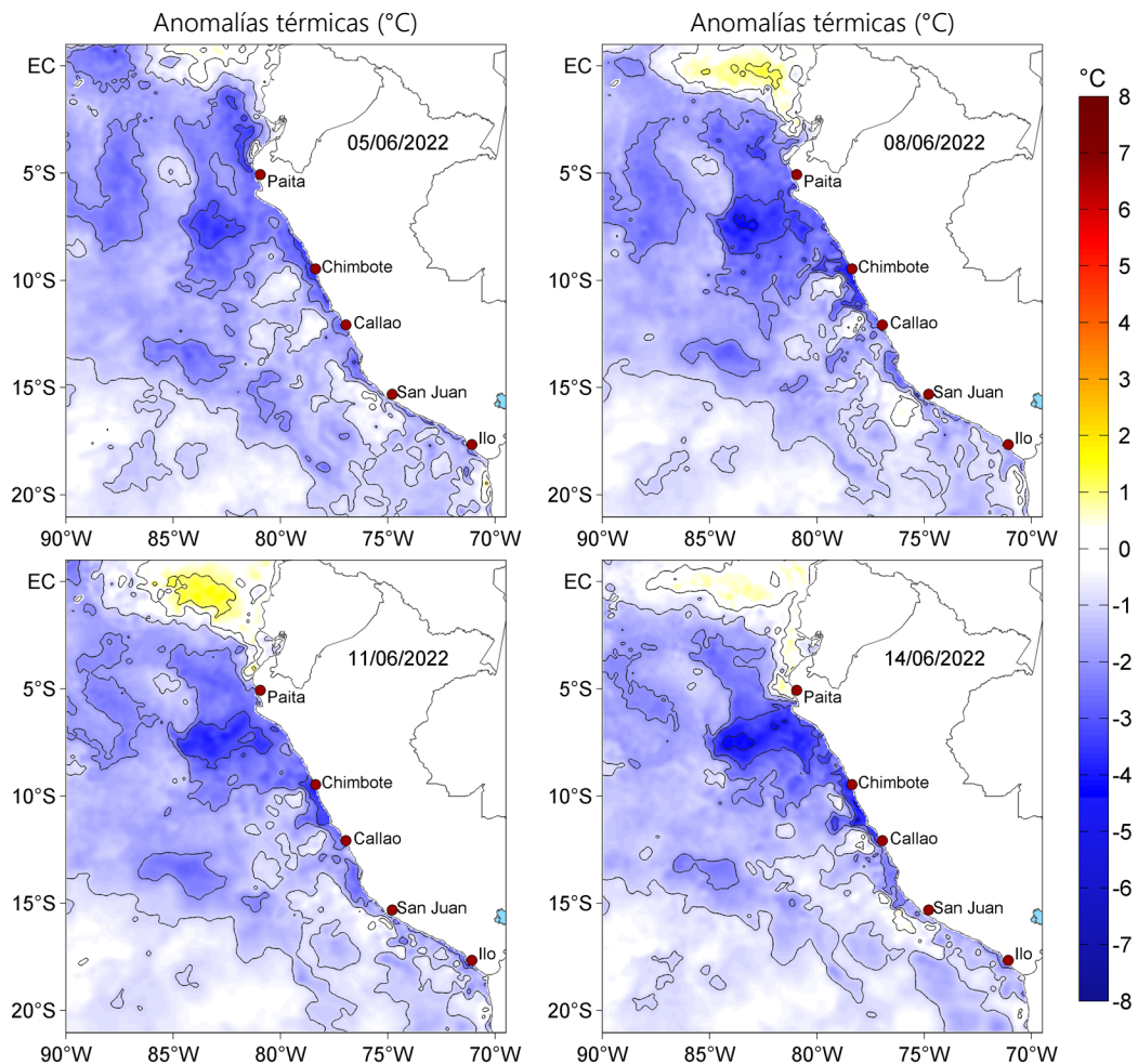
Figura 3. Anomalías de la temperatura superficial del mar (°C) para el 05, 08, 11 y 14 de junio de 2022. Las anomalías se calcularon respecto de la climatología para el periodo 2007-2016. Datos: OSTIA-UKMO-L4-GLOB-v2.0 (UK Met Office, 2012; Donlon et al, 2012).
