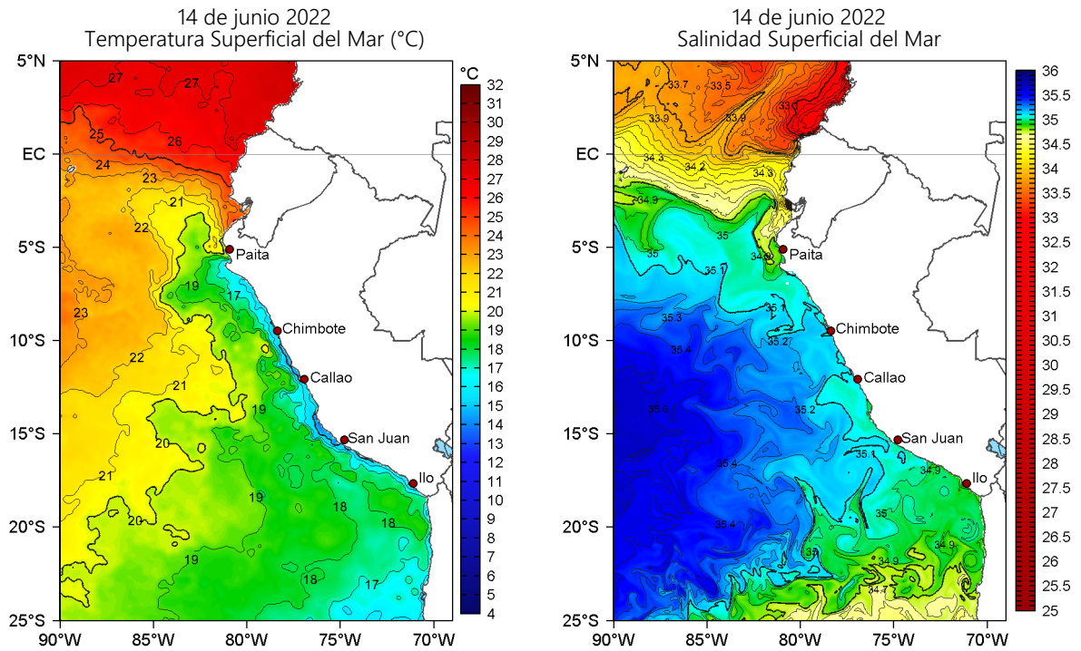
Figura 2. Temperatura superficial del mar (a la izquierda) y Salinidad superficial del mar (a la derecha) para el 14 de junio de 2022. Datos: OSTIA-UKMO-L4-GLOB-v2.0 (UK Met Office, 2012; Donlon et al, 2012) y Hybrid Coordinate Ocean Model v. GOFS 3.1 (HYCOM; Halliwell et al., 1998; 2000; Bleck, 2001), respectivamente.
