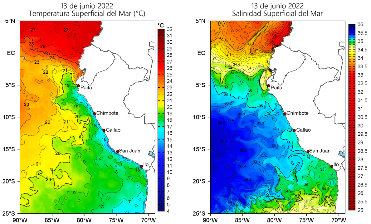
Figura 2. Temperatura superficial del mar (a la izquierda) y Salinidad superficial del mar (a la derecha) para el 13 de junio de 2022. Datos: OSTIA-UKMO-L4-GLOB-v2.0 (UK Met Office, 2012; Donlon et al, 2012) y Hybrid Coordinate Ocean Model v. GOFS 3.1 (HYCOM; Halliwell et al., 1998; 2000; Bleck, 2001), respectivamente.
