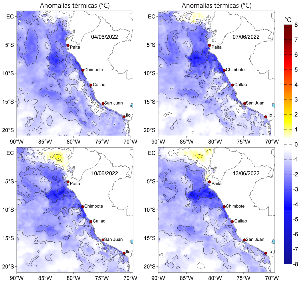
Figura 3. Anomalías de la temperatura superficial del mar (°C) para el 04, 07, 10 y 13 de junio de 2022. Las anomalías se calcularon respecto de la climatología para el periodo 2007-2016. Datos: OSTIA-UKMO-L4-GLOB-v2.0 (UK Met Office, 2012; Donlon et al, 2012).
