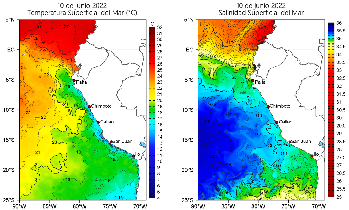
Figura 2. Temperatura superficial del mar (a la izquierda) y Salinidad superficial del mar (a la derecha) para el 10 de junio de 2022. Datos: OSTIA-UKMO-L4-GLOB-v2.0 (UK Met Office, 2012; Donlon et al, 2012) y Hybrid Coordinate Ocean Model v. GOFS 3.1 (HYCOM; Halliwell et al., 1998; 2000; Bleck, 2001), respectivamente.
