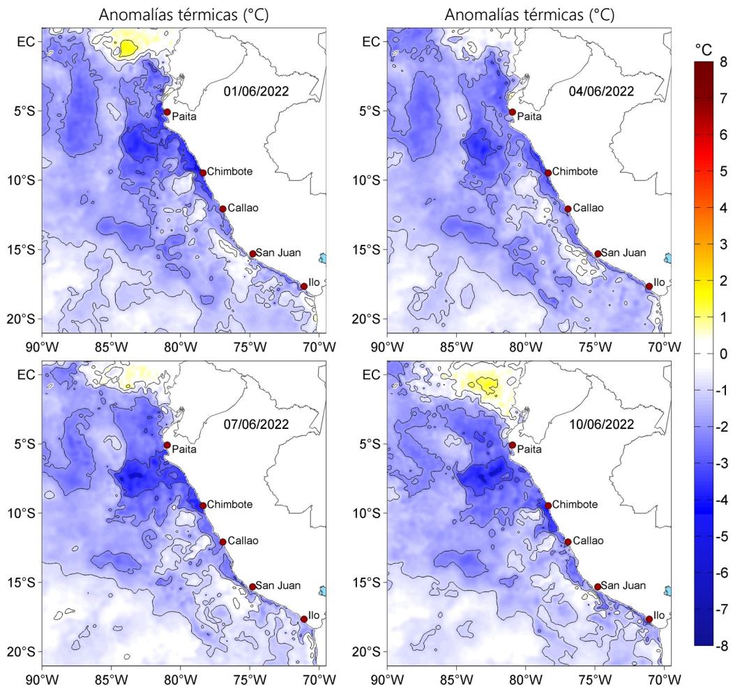
Figura 3. Anomalías de la temperatura superficial del mar (°C) para el 01, 04, 07 y 10 de junio de 2022. Las anomalías se calcularon respecto de la climatología para el periodo 2007-2016. Datos: OSTIA-UKMO-L4-GLOB-v2.0 (UK Met Office, 2012; Donlon et al, 2012).
