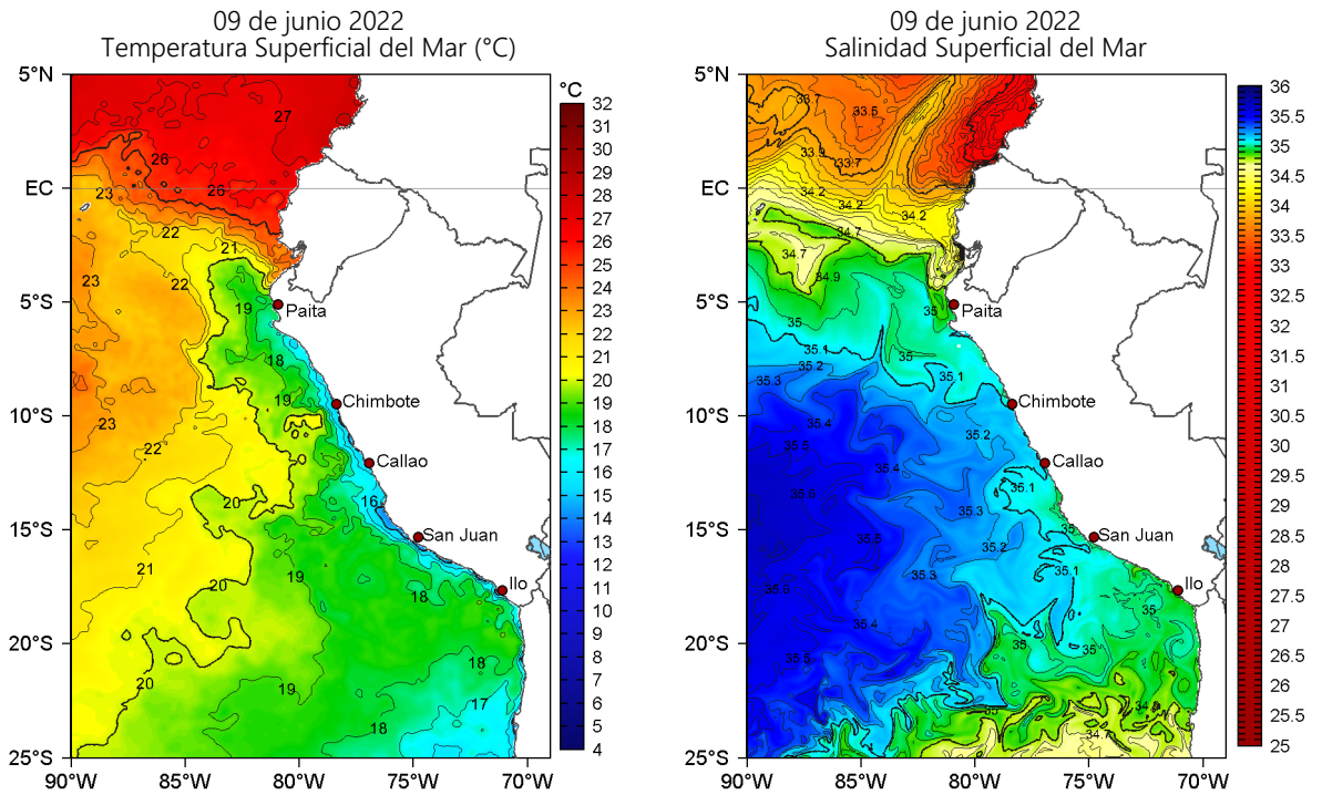
Figura 2. Temperatura superficial del mar (a la izquierda) y Salinidad superficial del mar (a la derecha) para el 09 de junio de 2022. Datos: OSTIA-UKMO-L4-GLOB-v2.0 (UK Met Office, 2012; Donlon et al, 2012) y Hybrid Coordinate Ocean Model v. GOFS 3.1 (HYCOM; Halliwell et al., 1998; 2000; Bleck, 2001), respectivamente.
