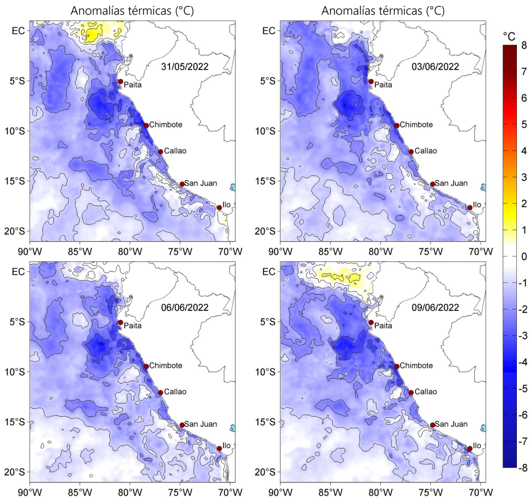
Figura 3. Anomalías de la temperatura superficial del mar (°C) para el 31 de mayo, así como para el 03, 06 y 09 de junio de 2022. Las anomalías se calcularon respecto de la climatología para el periodo 2007-2016. Datos: OSTIA-UKMO-L4-GLOB-v2.0 (UK Met Office, 2012; Donlon et al, 2012).
